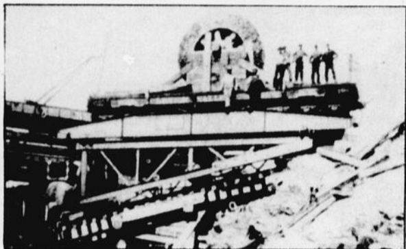
Plate-forme funiculaire servant à descendre les équipements lourds lors de la construction de la seconde centrale de la Shawinigan Water and Power.
