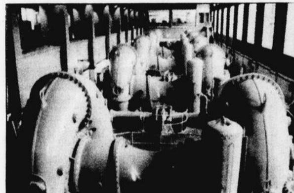
Groupes turbo-alternateurs horizontaux installés dans la centrale II en opération.
