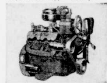
LE NOUVEAU V-6 351 GMC allie à l'économie d'un 6-cylindres la performance d'un robuste moteur en V. Puissance de 180 cv—couple de 312 lb/pi—3400 t/m. Facilité sur les modèles des séries C970 et C980.
