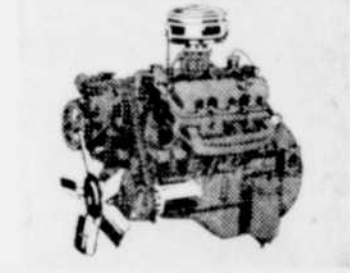
LE PUISSANT V-6 401 GMC. Puissance de 210 cv—couple de 377 lb/pi—3400 t/m. Idéal pour les camions ayant un PBV de 25,000—32,000 lb.
