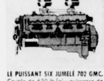
LE PUISSANT SIX JUMELÉ 702 GMC. Couple de 630 lb/pi—puissance de 275 cv—2400 t/m. Ce moteur 6 jumelés est le plus puissant moteur à essence qui soit offert comme équipement standard.
