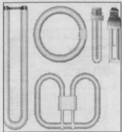
LAMPES FLUORESCENTES - Il existe diverses formes de lampes fluorescentes, notamment en U, circulaires et compactes.
