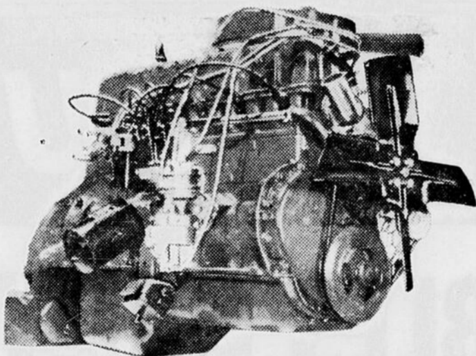
Moteur "Torque Command" à vilebrequin supporté sur 7 paliers—le remarquable nouveau six-cylindres qui a le rendement d'un huit! Facultatif sur tous les modèles Rambler 1965.
