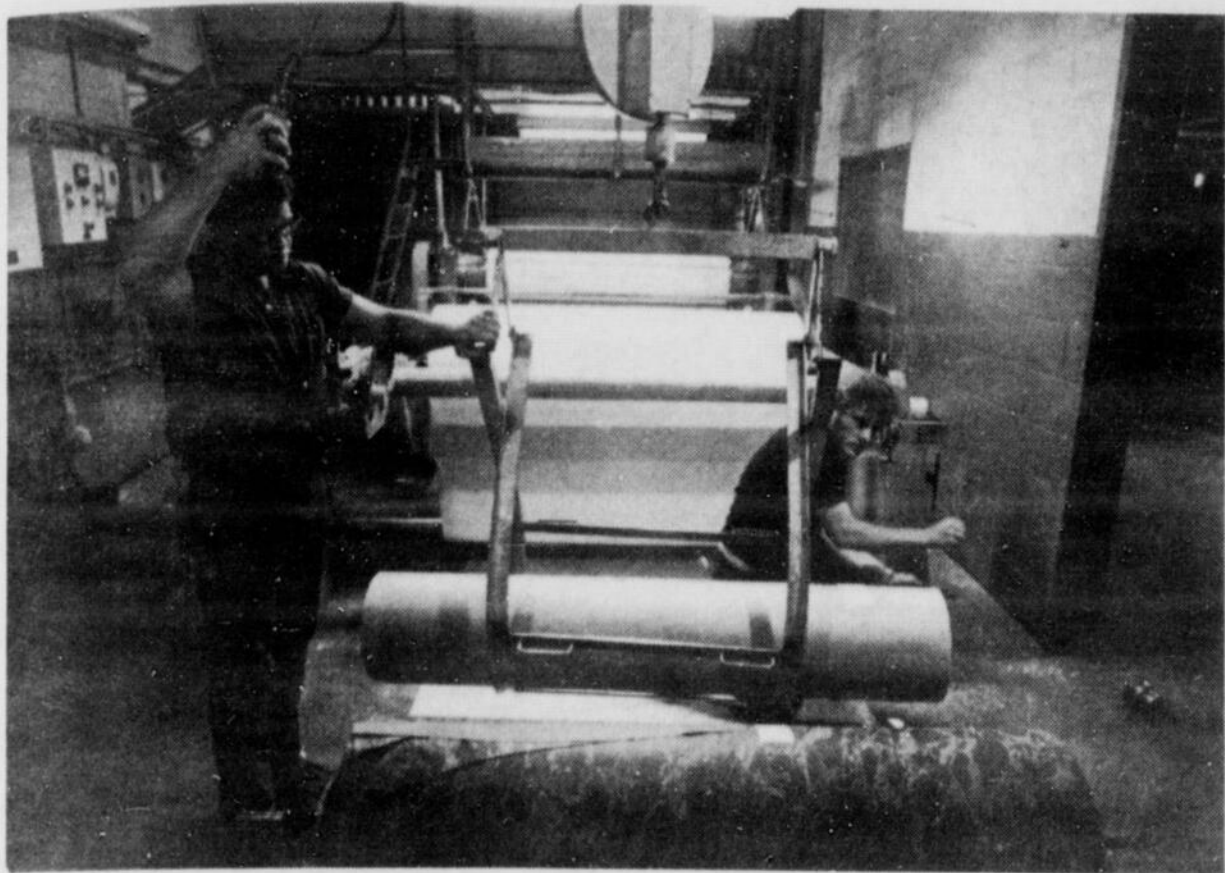
L'une des premières opérations dans la production des panneaux laminés de "Formica" est l'imprégnation du papier avec des résines mélamine. De l'autre côté de cette machine, le papier sortira, coupé en longueurs données, et séché.
