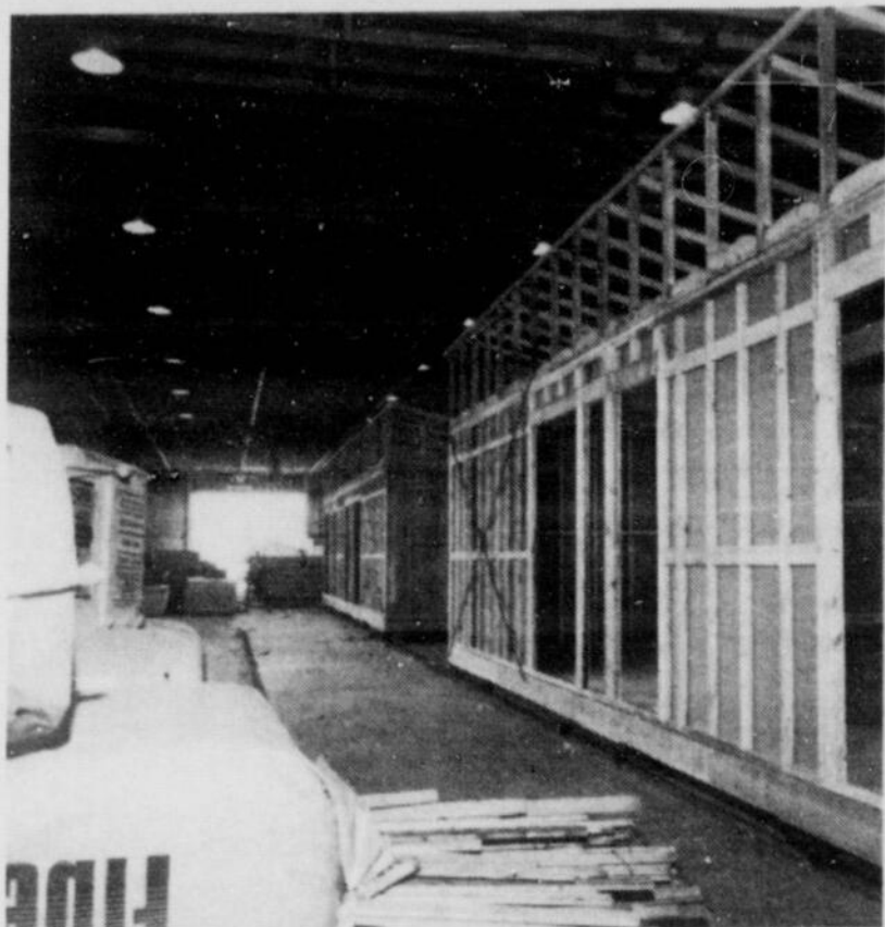
Charpentes de maisons usinées par section.
