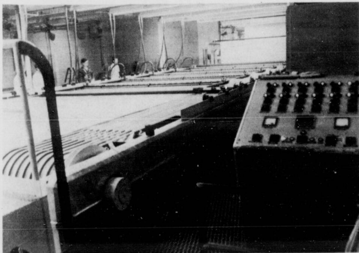
Voici la machine qui sert au nouveau procédé "Zimmer" dans la fabrication des tapis Ozite imprimés.
