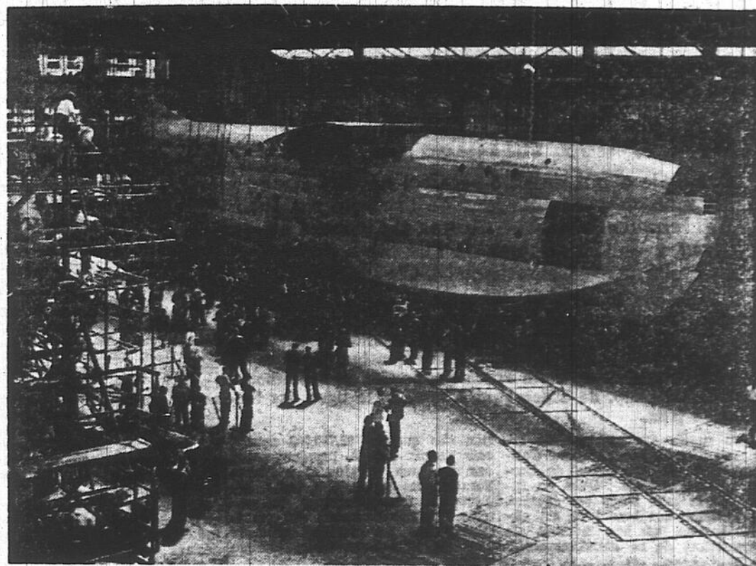
La plus grande coque jamais construite pour un avion est ce châssis géant de la catégorie des navires-volants "Princess" actuellement construite à Wight, Angleterre. Elle pèse cent quarante tonnes avec une expansion d'ailes de 240 pieds. Elle a cinquante-cinq pieds de haut et pourra accommoder cent passagers. La coque telle qu'on la voit actuellement est prête pour l'installation des moteurs.
