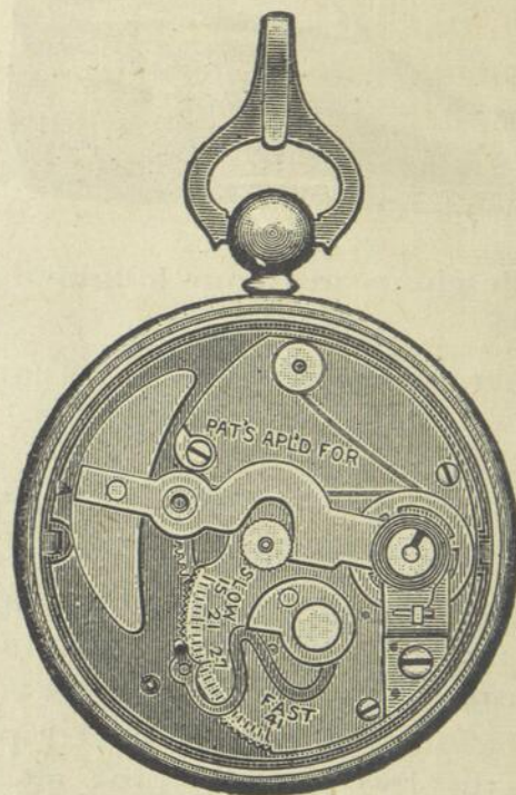
Le mécanisme du pedomètre.
