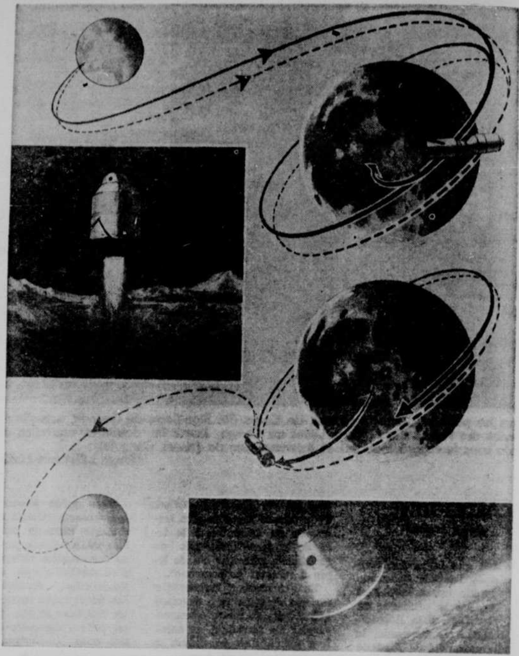
Dans le cas de la technique de rendez-vous en orbite lunaire, le Saturn C-5 mettrait en orbite autour de la Lune une charge de 90,000 livres. De cette orbite lunaire, un autre appareil effectuerait le voyage à la surface de la Lune.
