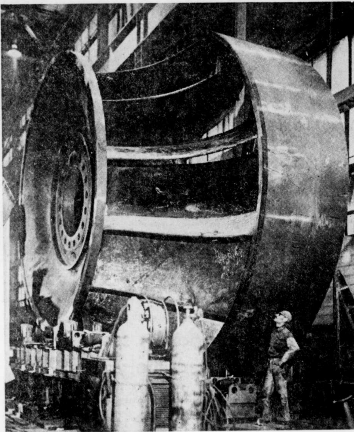
La société Dominion Engineering Works, de Lachine, est un des rares manufacturiers au monde à pouvoir produire des turbines de plus de 800 mégawatts de puissance. Cette turbine en cours de fabrication aux usines de Lachine n'est pas destinée au Brésil, mais aux Etats-Unis. Celles qui doivent équiper la centrale brésilienne d'Itaipu sont encore plus grosses.
