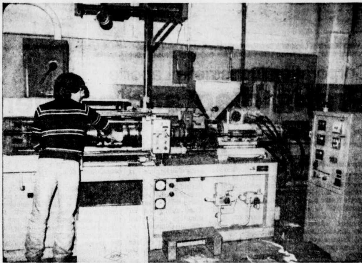
Un élève procédant aux étapes de pose d'un moule et réglage mécanique de la machine.
