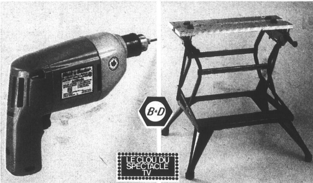
Voyez les spéciaux de télé de Black & Decker... pour des cadeaux idéals! Perceuse réversible de 3/8" à vitesse variable. Avec vitesse blocable par gâchette; cordon amovible. Capacité: acier 3/8", bois 3/4". N° 7190-04. 34 88 Workmate Deluxe portatif: à la fois un grand étau et un chevalet de sciage. Se plie pour le rangement. Leviers 2 positions; chevilles pivotantes. #79-005 56 88
