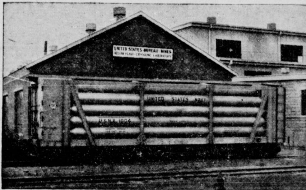
Wagon-réservoir naval spécialement construit pour le transport de l'hélium.
