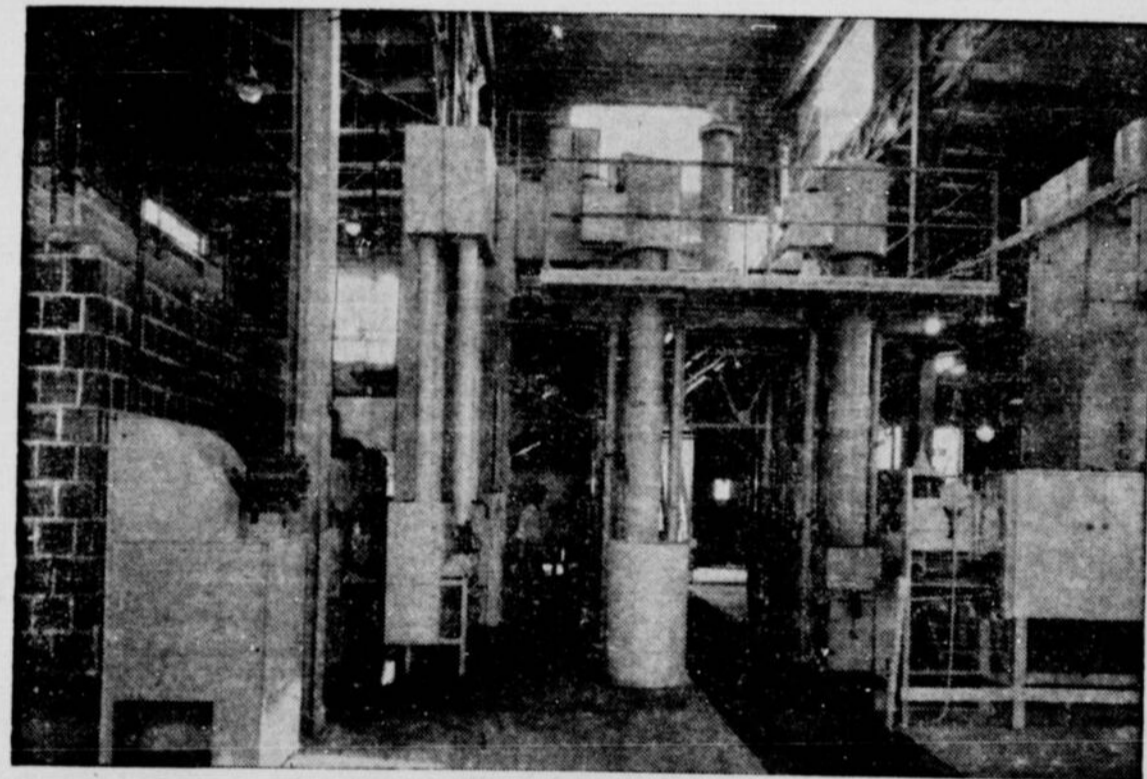
C'est à travers cette série de tubes et de réservoirs que l'hélium est isolé sous forme de gaz des autres éléments qui constituent le gaz naturel porteur d'hélium. Cette opération est faite à des températures plus basses que 300 degrés Fahrenheit à l'usine d'Amarillo, Texas.
