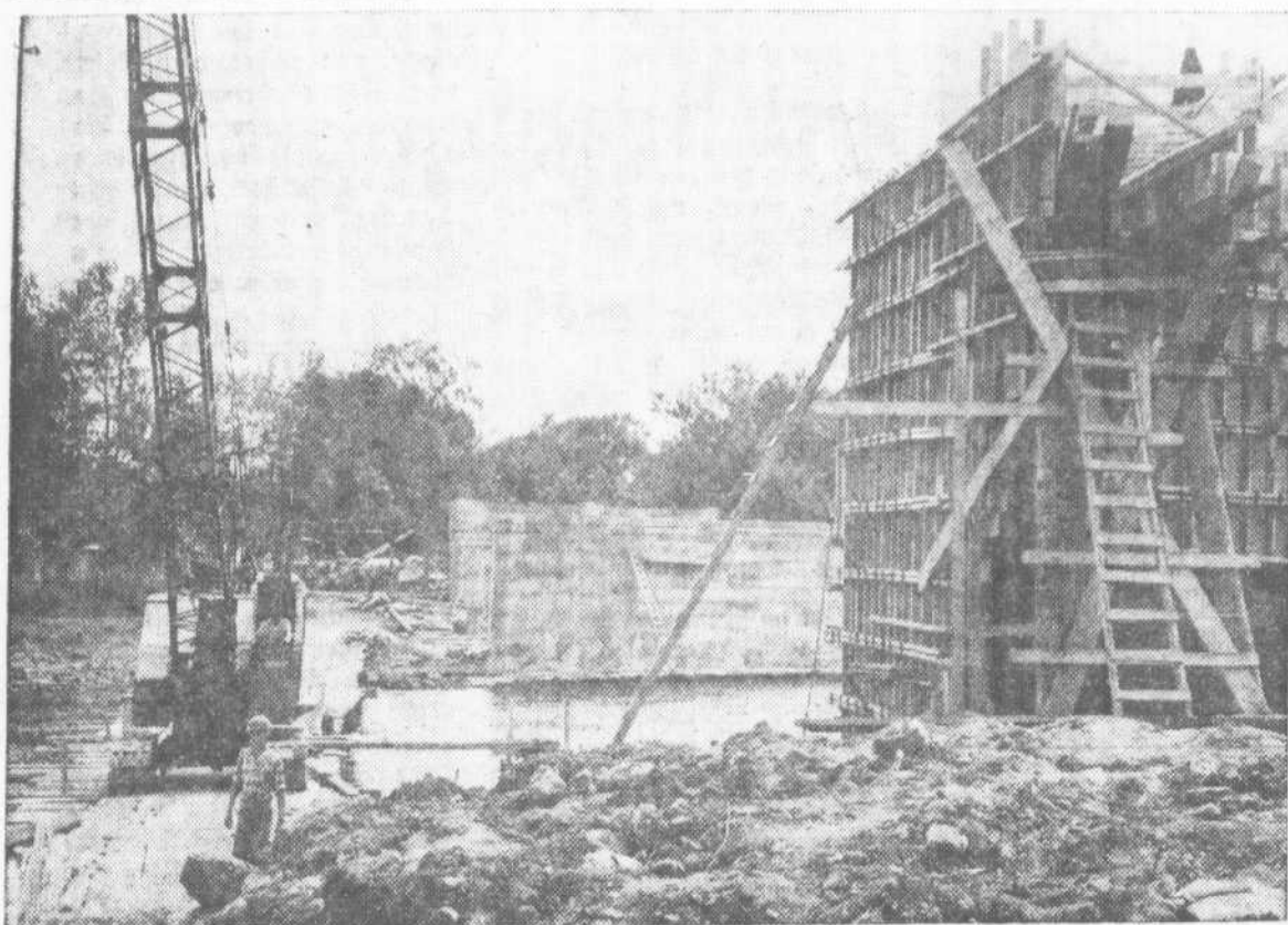
UNE PARTIE DES TRAVAUX DU PONT DE TERREBONNE dans Ville St-François. On voit ici la première partie reliant la rive sud à l'île St-Jean. Le pont sera construit entièrement en béton armé et aura un peu plus de 1,000 pieds de longueur. Les travaux se poursuivent à un rythme accéléré et doivent être terminés en août 1964.
