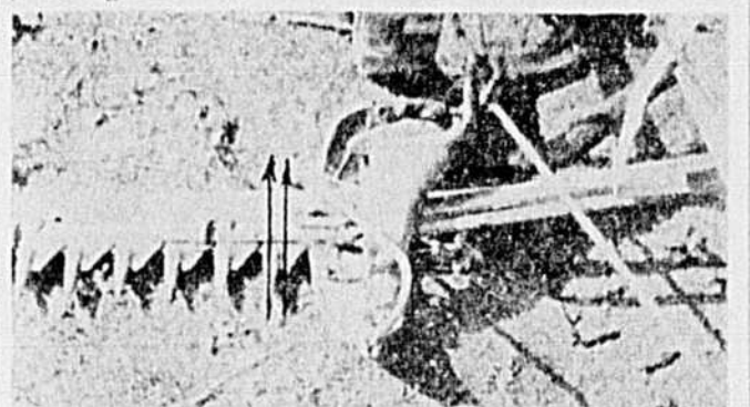
● MAUVAIS ENGOUGEAGE : les pointes des couteaux et les doigts ne sont pas alignés.
