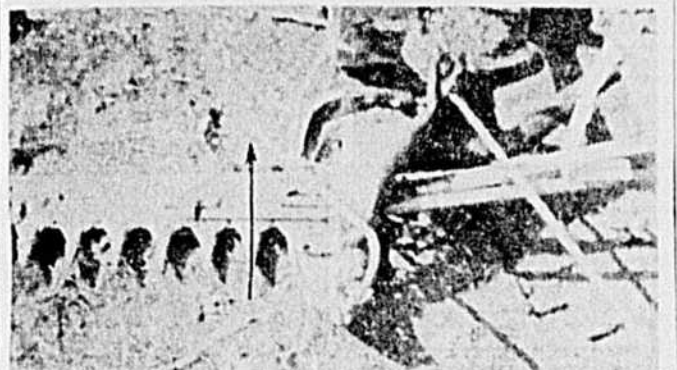
● MODÈLE D'ENGOUGEAGE PARFAIT : la pointe des couteaux centrée bien au milieu des doigts lorsque la bielle est au bout de sa course.
