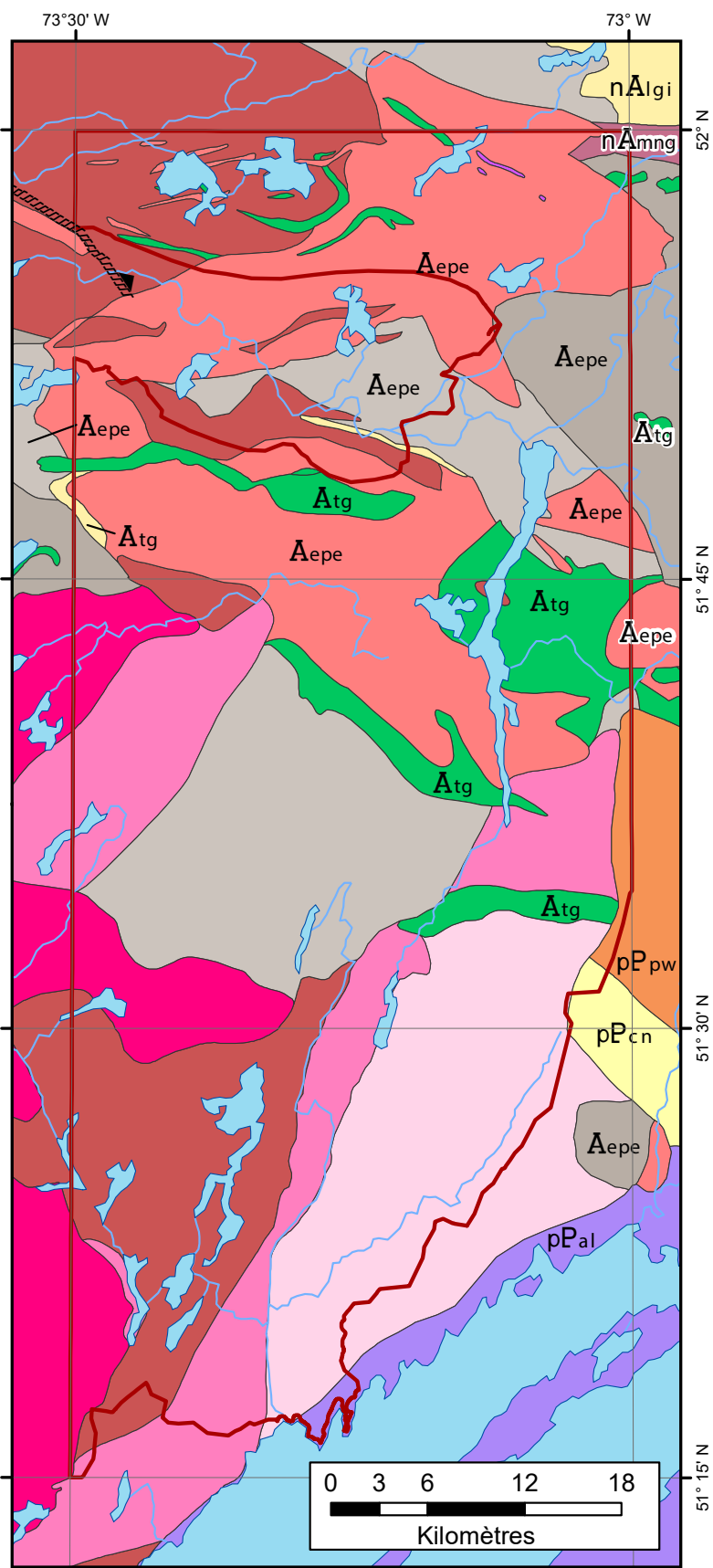
FIGURE 2 – Carte géologique du secteur d'étude modifiée de Roy (2023), Chown (1971) et Chown et Caty (1973)
