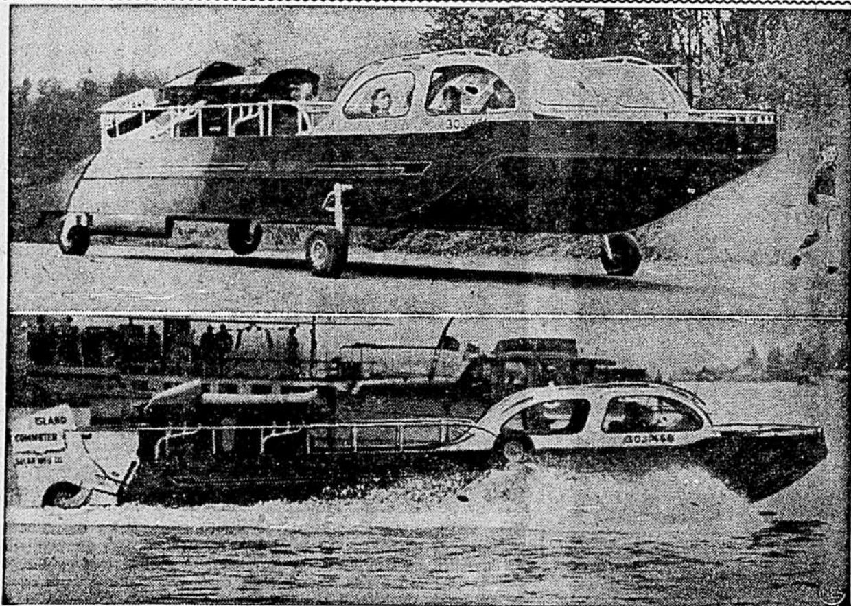
SUR TERRE ET SUR MER. — Tony Sulak a réalisé un rêve: un véhicule automobile qui peut rouler sur la terre ferme et qui peut aussi devenir un imposant yacht de plaisance. L'auto-yacht mesure 32 pieds de longueur et a coûté $24,000 à Sulak. L'appareil amphibie est mis en mouvement par des hélices d'avion, placées à l'arrière, et actionnées par deux moteurs. Dans la photo du bas, on voit l'appareil faisant une excursion d'essai sur le lac Washington.
