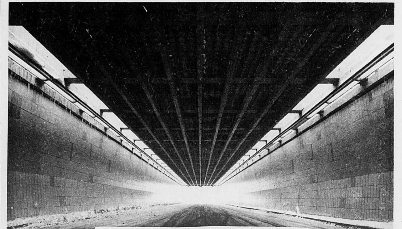
A chacun des portails, un brise-soleil formé d'alvéoles d'une profondeur de 24 pouces atténue progressivement la lumière du jour pour passer à une intensité de douze pieds-bougies, 1,000 pieds à l'intérieur du tunnel.
