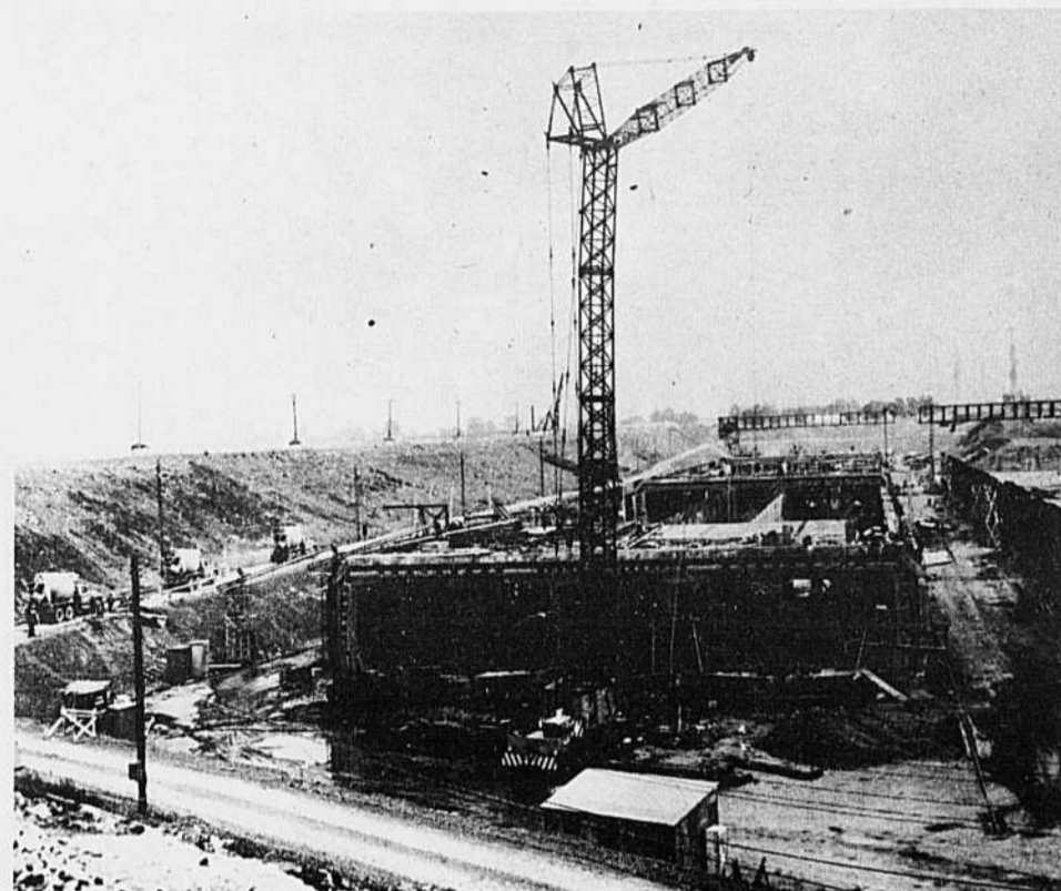
A l'automne 1964, les ouvriers s'affairaient à la construction des sept éléments du tunnel Louis-Hippolyte Lafontaine. Les deux tubes de circulation, dont on aperçoit les contours sur la photo, offrent chacun trois pistes de roulement d'une largeur totale de 38 pieds.
