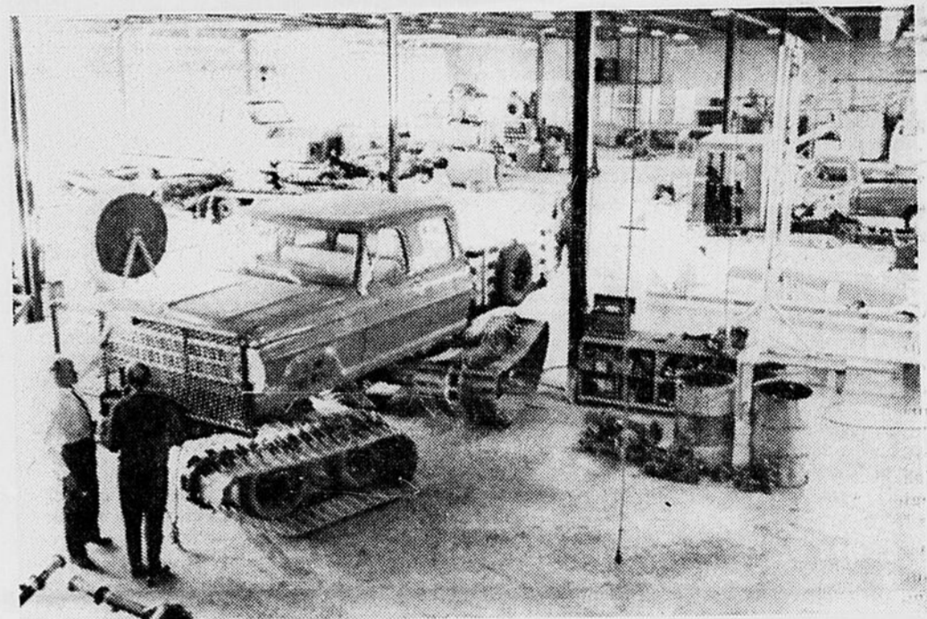
Véhicules à traction fabriqués à la Foremost Developments Ltd., à Edmonton.
