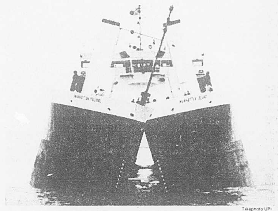
La North American Trailing Company vient de faire l'acquisition du deuxième navire dragueur à coque ouvrante au monde. D'une longueur de 281 pieds, le "Manhattan Island" peut décharger 3,600 verges cubes de terre en 40 secondes, grâce à l'ouverture de la coque jusqu'à un maximum de 16 pieds et demi.
