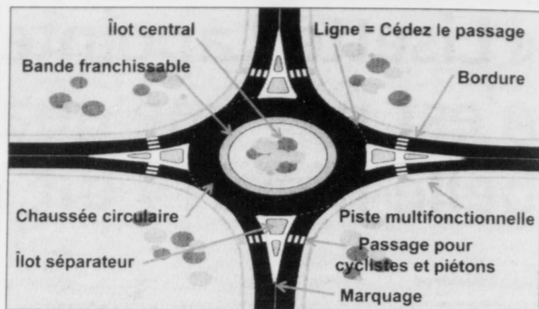
Un carrefour giratoire est un aménagement comprenant une chaussée entourant un îlot central. La circulation s'y fait à sens unique, dans le sens contraire des aiguilles d'une montre. Les usagers qui veulent s'engager dans le carrefour doivent céder le passage aux piétons, aux cyclistes et aux véhicules qui y circulent déjà. — PLAN FOURNI PAR LE MINISTÈRE DES TRANSPORTS
