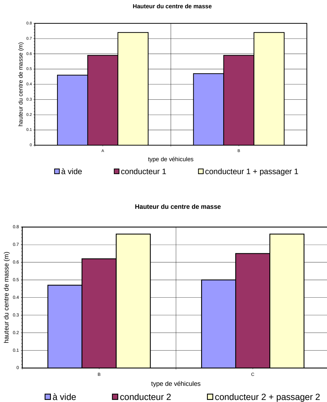
Figure 10a: Hauteur du centre de masse en fonction du nombre de passagers.
