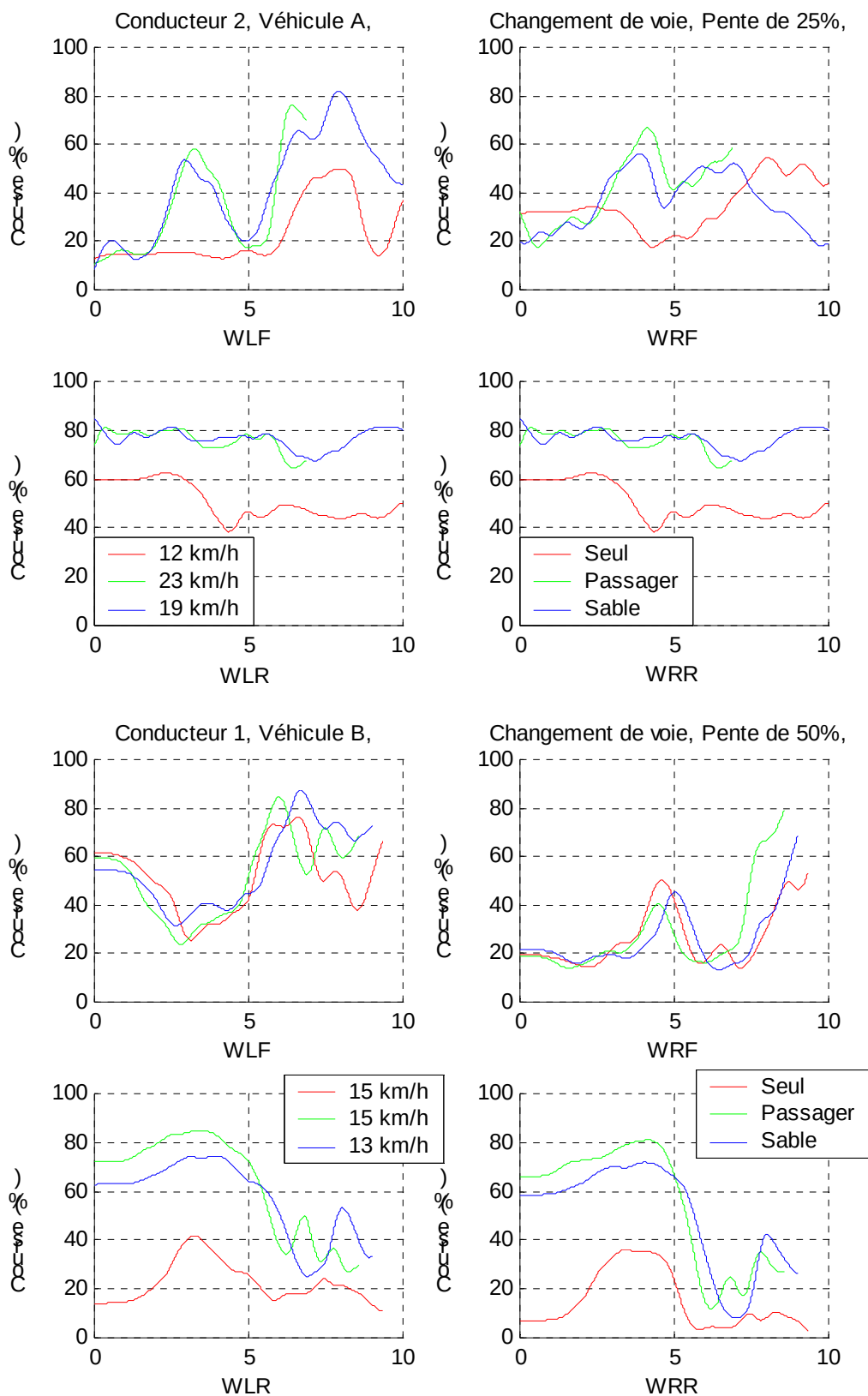
Figure 35: Transfert de charge durant un changement de voie
