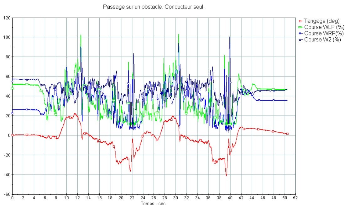
Figure 38a: Courses des suspensions lors d'un impact sur un obstacle. (Conducteur seul)
