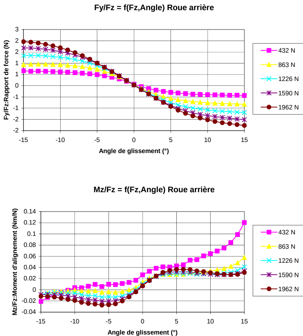
Figure 19: Forces latérales et moments d'alignement aux roues avant et arrière.
