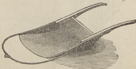
GRATTOIR DE CHEMIN. —Le grattoir de chemin No. 2 est tout en fonte, canton en fer forgé et manches de bois. Prix, $9.00.
