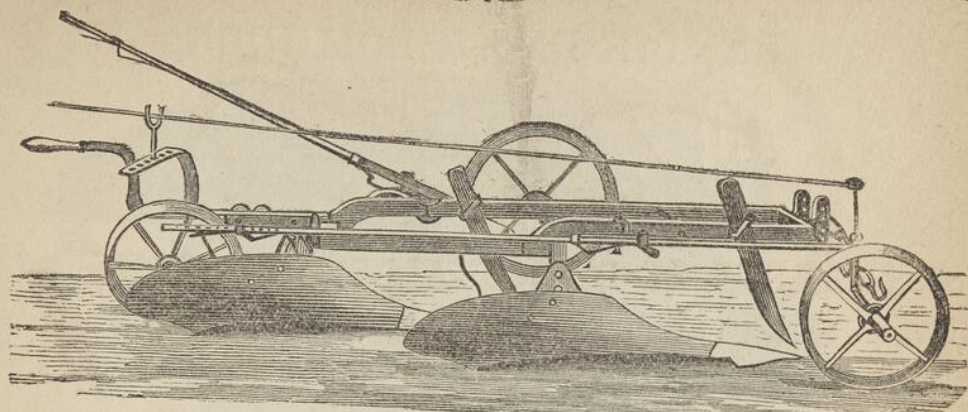
Charrue à double sillons, en fer forgé, prenant de deux à quatre chevaux. Prix de $50.00 à $75.00.
