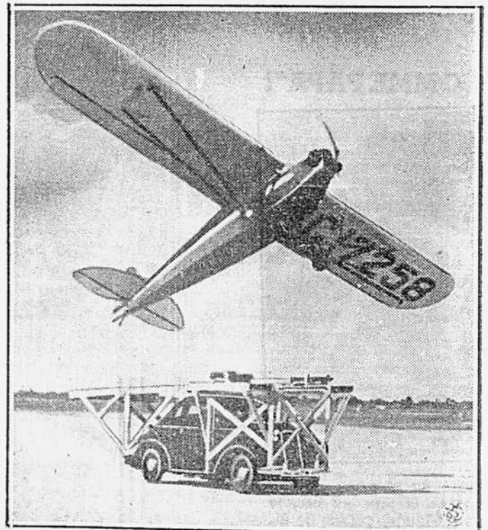
Voici un avion s'élevant gracieusement d'une auto filant à près de cent milles à l'heure. Cette façon de décoller convient sur les aéroports qui ont peu d'espace.
