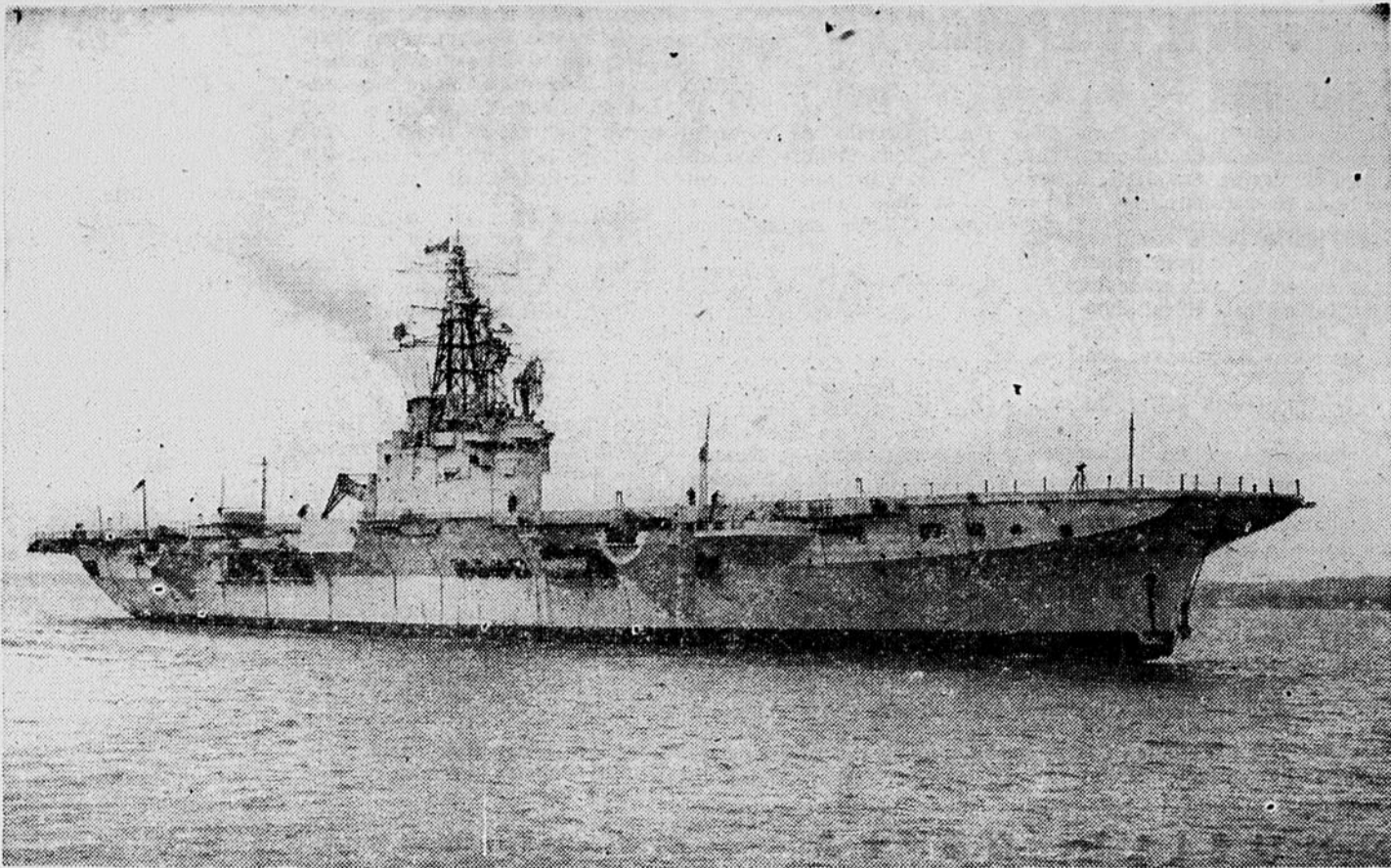
NOUVEAU PORTE-AVION DU CANADA — Navigant sous sa propre puissance pour la première fois, le porte-avion Bonaventure descend le bras de mer de Belfast pour entreprendre ses épreuves en mer. Construit à Belfast, Irlande du Nord, le Bonaventure sera armé le 17 janvier prochain dans la MRC.
