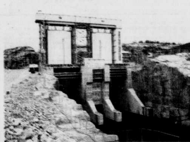
Vannes de l'évacuateur de la Rupert (2008)
