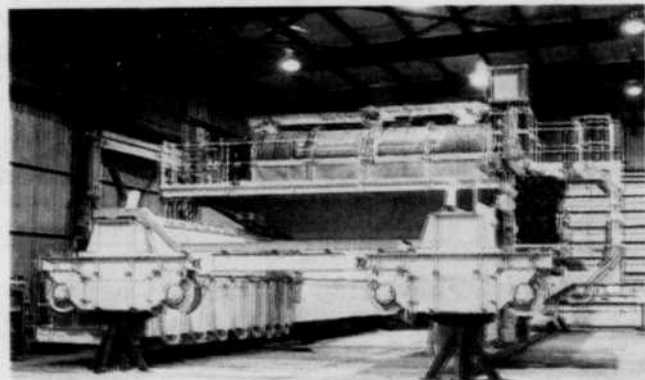
Pont roulant de 210 tonnes métriques (2009)
