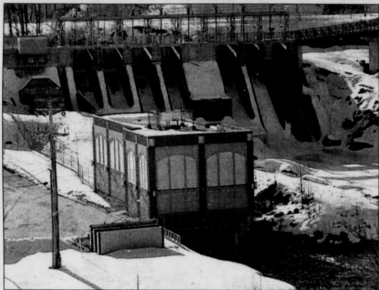
La centrale hydroélectrique Saint-Damase est située sur la rivière Aux Sables. Elle appartient à Hydro-Jonquière et est d'une capacité de 3900 kilowatts.
