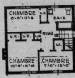
PREMIER PLANCHER
