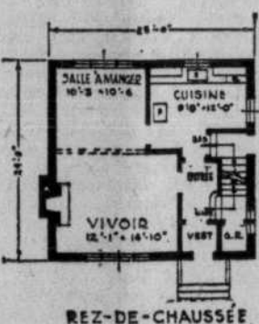
REZ-DE-CHAUSSEE
