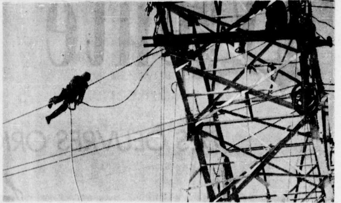
Poseurs de lignes qualifiés et forcément acrobates, des employés de Checo Enterprises Inc., compagnie qui construit la ligne Manicouagan-Montréal de 735,000 volts pour l'Hydro-Québec, sont ici photographiés à 100 pieds du sol. A gauche, un homme pose une bride qui soutiendra 1,600 pieds de câble d'aluminium renforcé Alcan.
