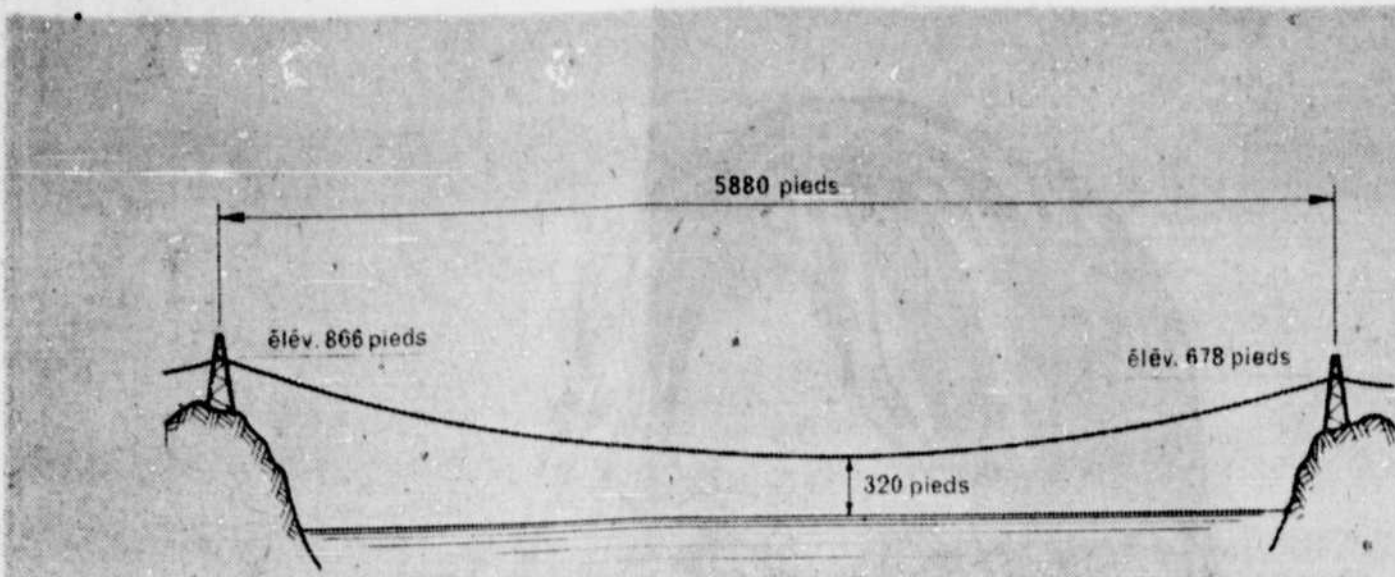
PREMIÈRE LIGNE DE TRANSPORT DE 735.000 VOLTS
