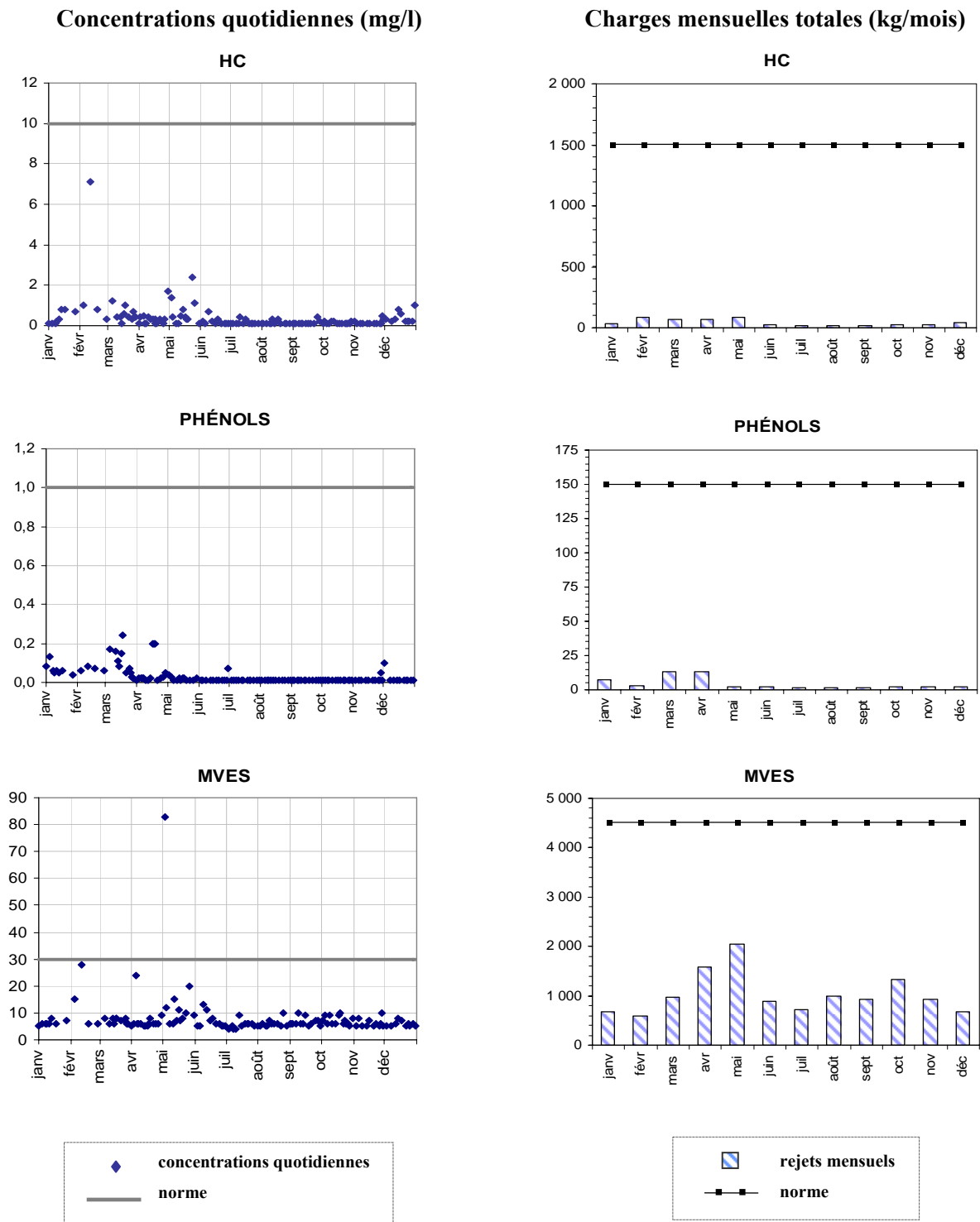
Figure B - 3 Concentrations quotidiennes et charges mensuelles totales dans l'effluent d'eaux pluviales de Pétro-Canada en 2007 en comparaison des normes
