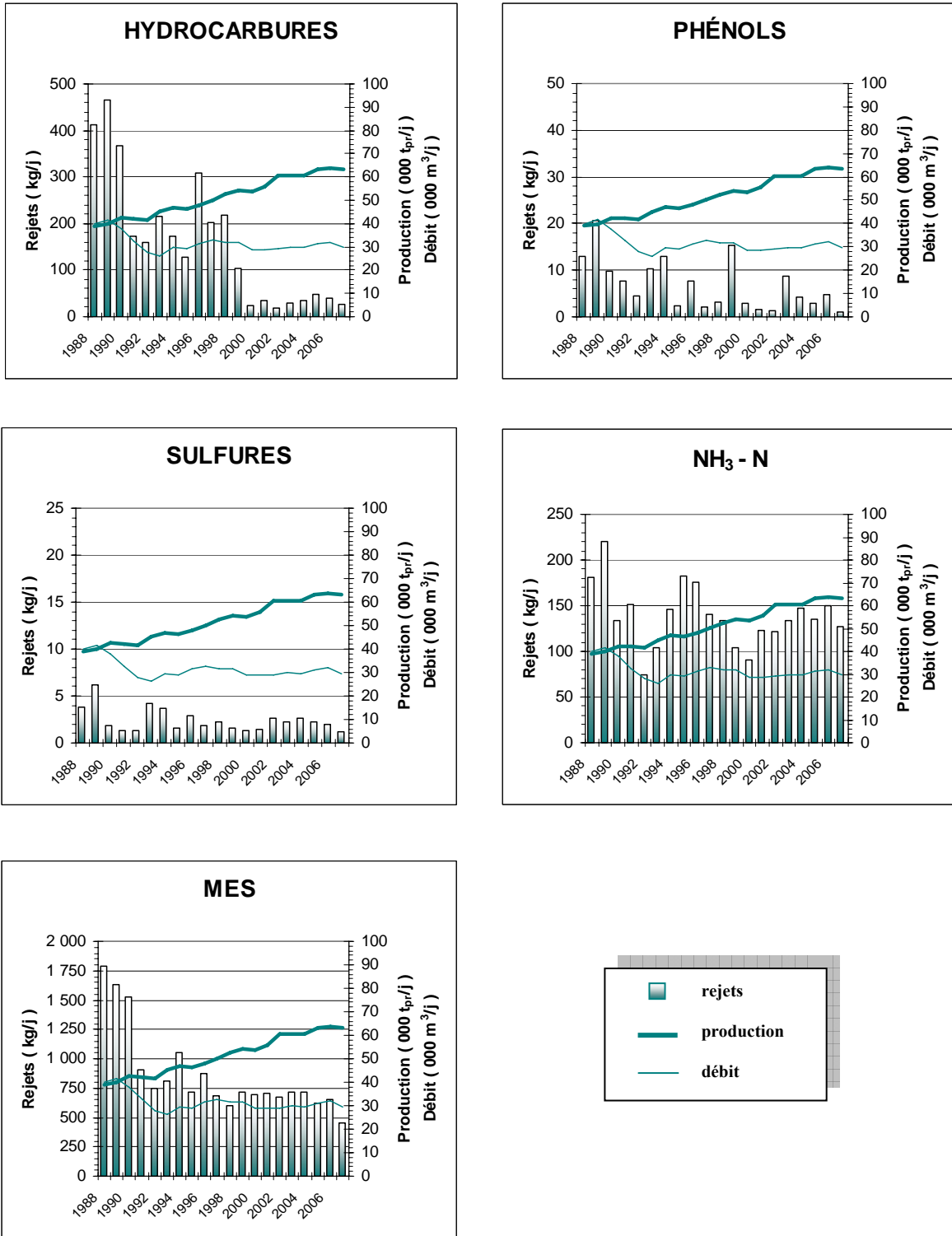
Figure 6 Évolution des charges des contaminants normés dans les effluents d'eaux de procédé des raffineries québécoises, de la production et des débits quotidiens, de 1988 à 2007
