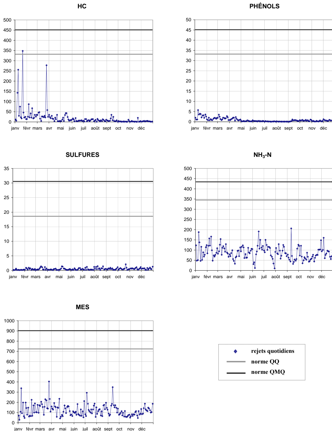
Figure B - 1 Charges quotidiennes dans l'effluent d'eaux de procédé de Pétro-Canada en 2007 en comparaison des normes (kg/j)
