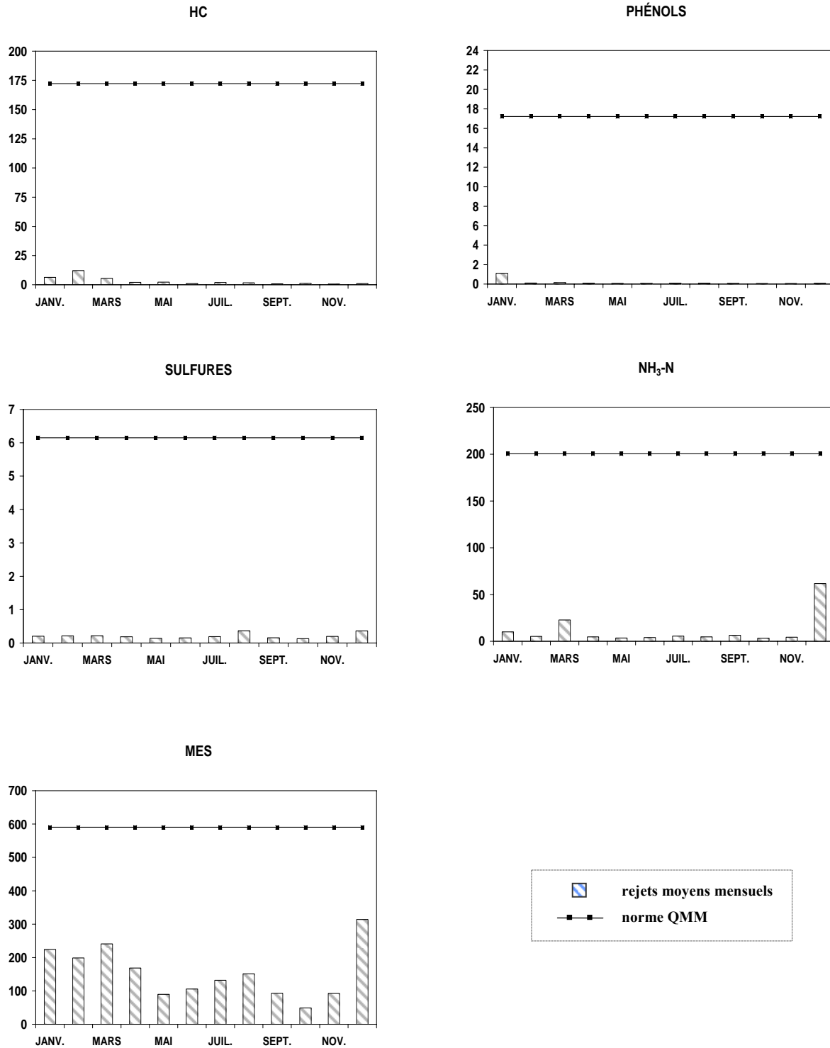
Figure B - 5 Charges moyennes dans l'effluent d'eaux de procédé de Shell Canada ltée en 2007 en comparaison des normes (kg/j)
