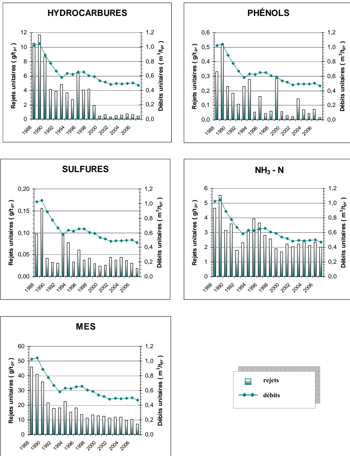
Figure 7 Évolution des charges unitaires des contaminants normés rejetés par les effluents d'eaux de procédé de l'ensemble des raffineries, de 1988 à 2007
