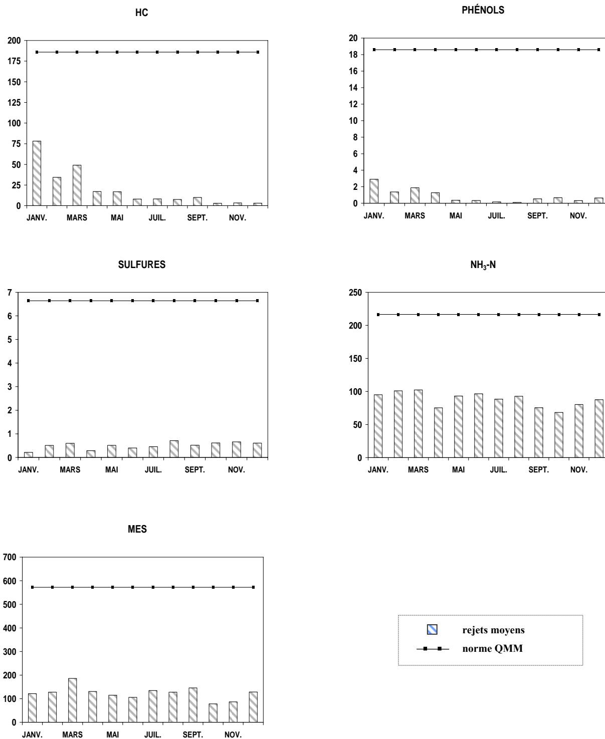
Figure B - 2 Charges moyennes dans l'effluent d'eaux de procédé de Pétro-Canada en 2007 en comparaison des normes (kg/j)
