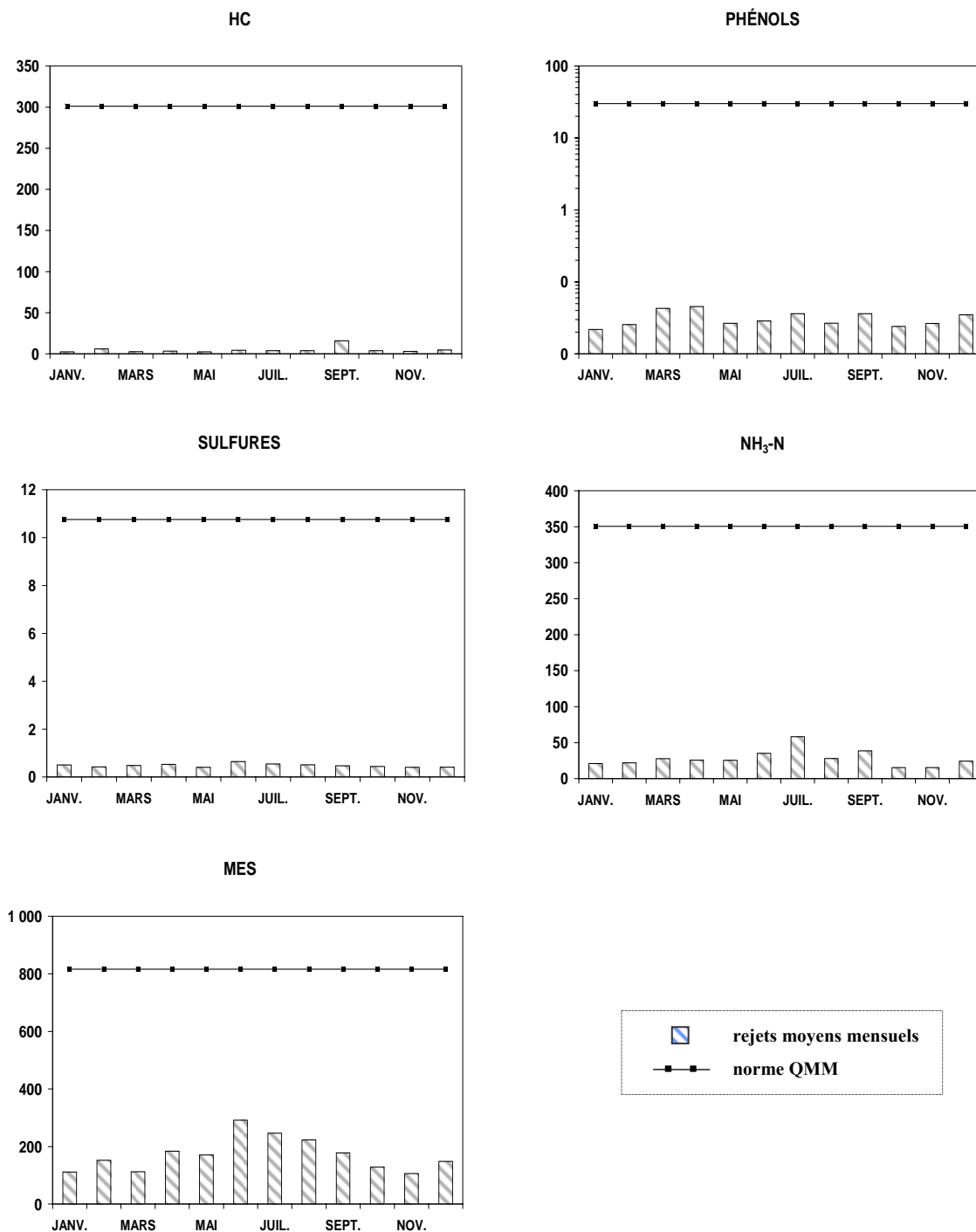
Figure B - 8 Charges moyennes dans l'effluent d'eaux de procédé d'Ultramar en 2007 en comparaison des normes (kg/j)
