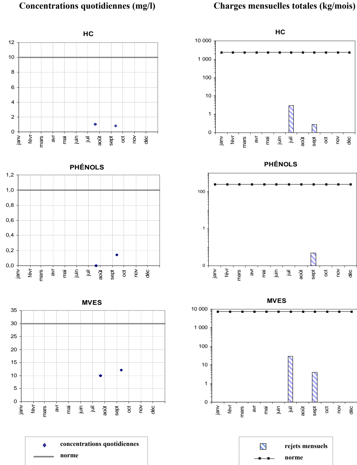
Figure B - 9 Concentrations quotidiennes et charges mensuelles totales dans l'effluent d'eaux pluviales d'Ultramar en 2007 en comparaison des normes
