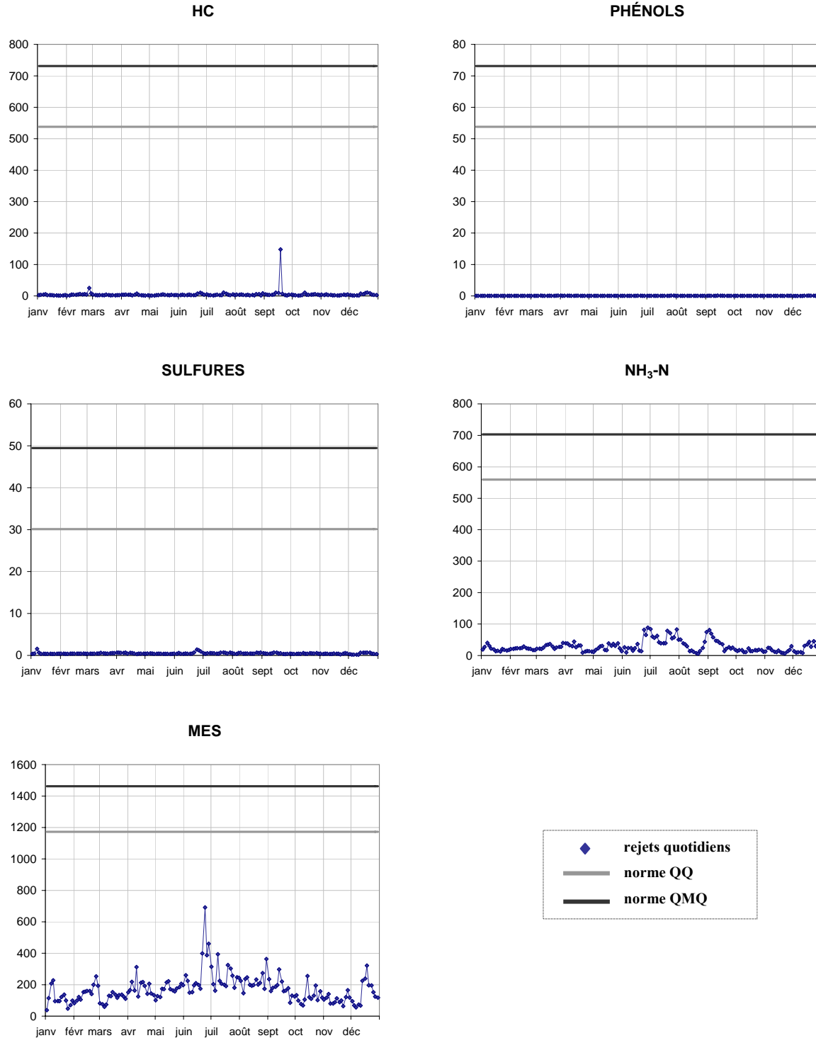
Figure B - 7 Charges quotidiennes dans l'effluent d'eaux de procédé d'Ultramar en 2007 en comparaison des normes (kg/j)
