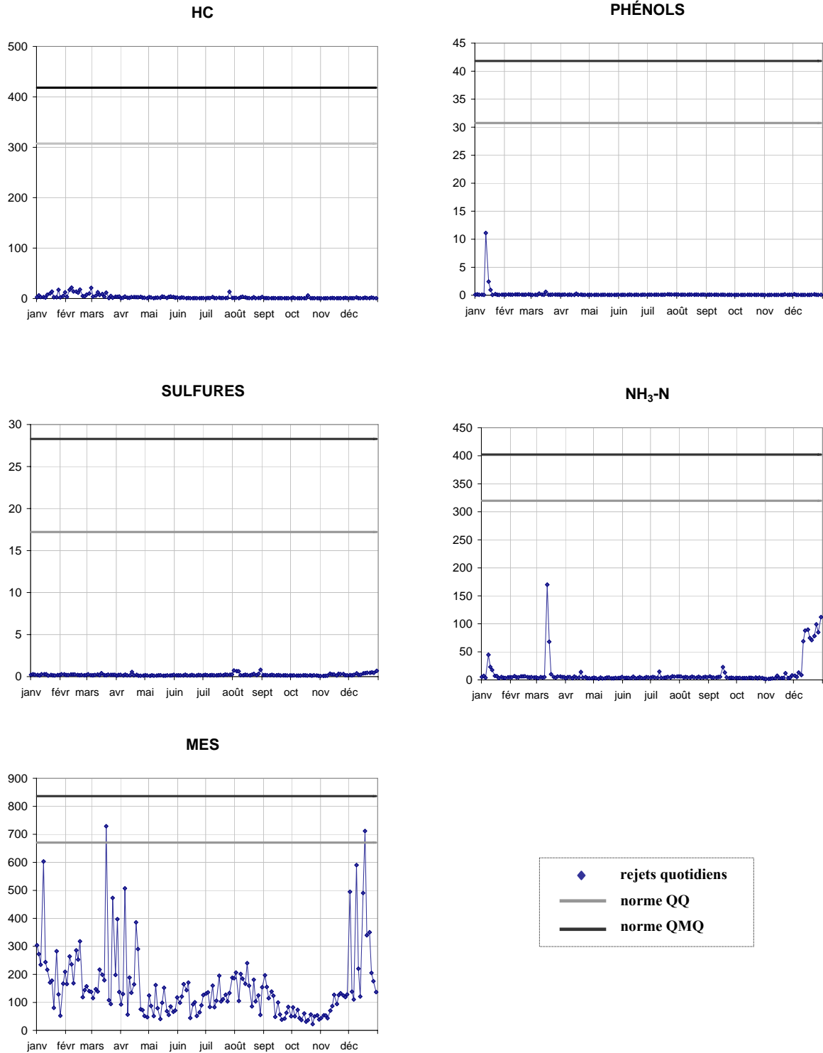
Figure B - 4 Charges quotidiennes dans l'effluent d'eaux de procédé de Shell Canada ltée en 2007 en comparaison des normes (kg/j)
