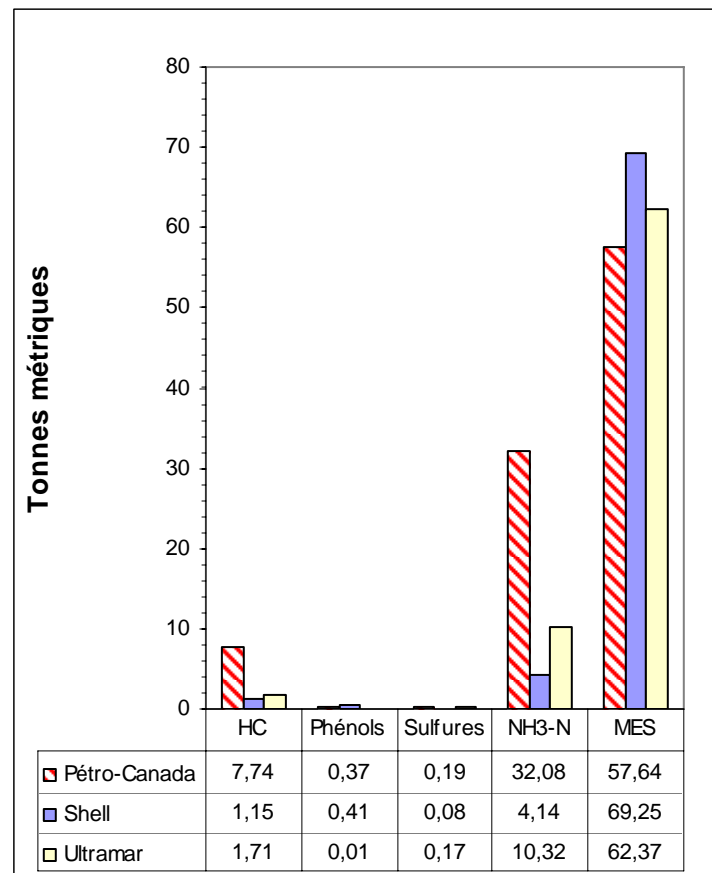
Figure 3 Charges totales des contaminants normés rejetés par chacune des raffineries en 2007 (t)
