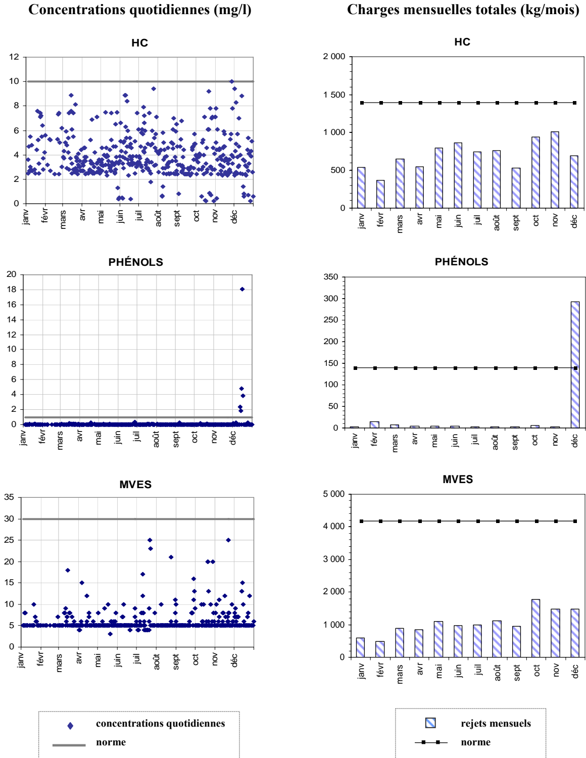
Figure B - 6 Concentrations quotidiennes et charges mensuelles totales dans l'effluent d'eaux pluviales de Shell Canada Ltée en 2007 en comparaison des normes
