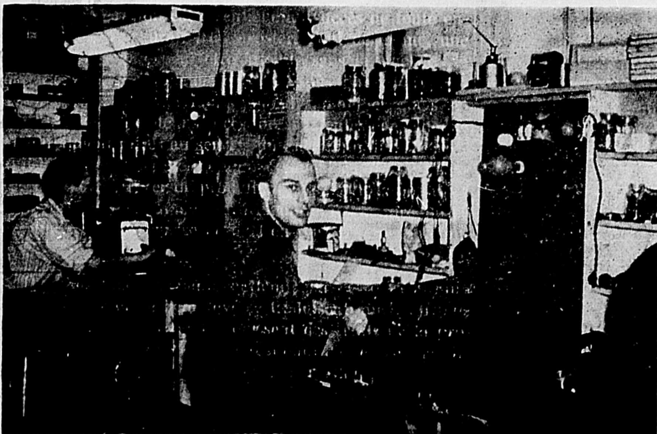
M. Guy Beaudoin, à gauche, répare un accessoire électrique. M. Raymond Noël refait le filage d'une armature de générateur servant à la soudure électrique.
