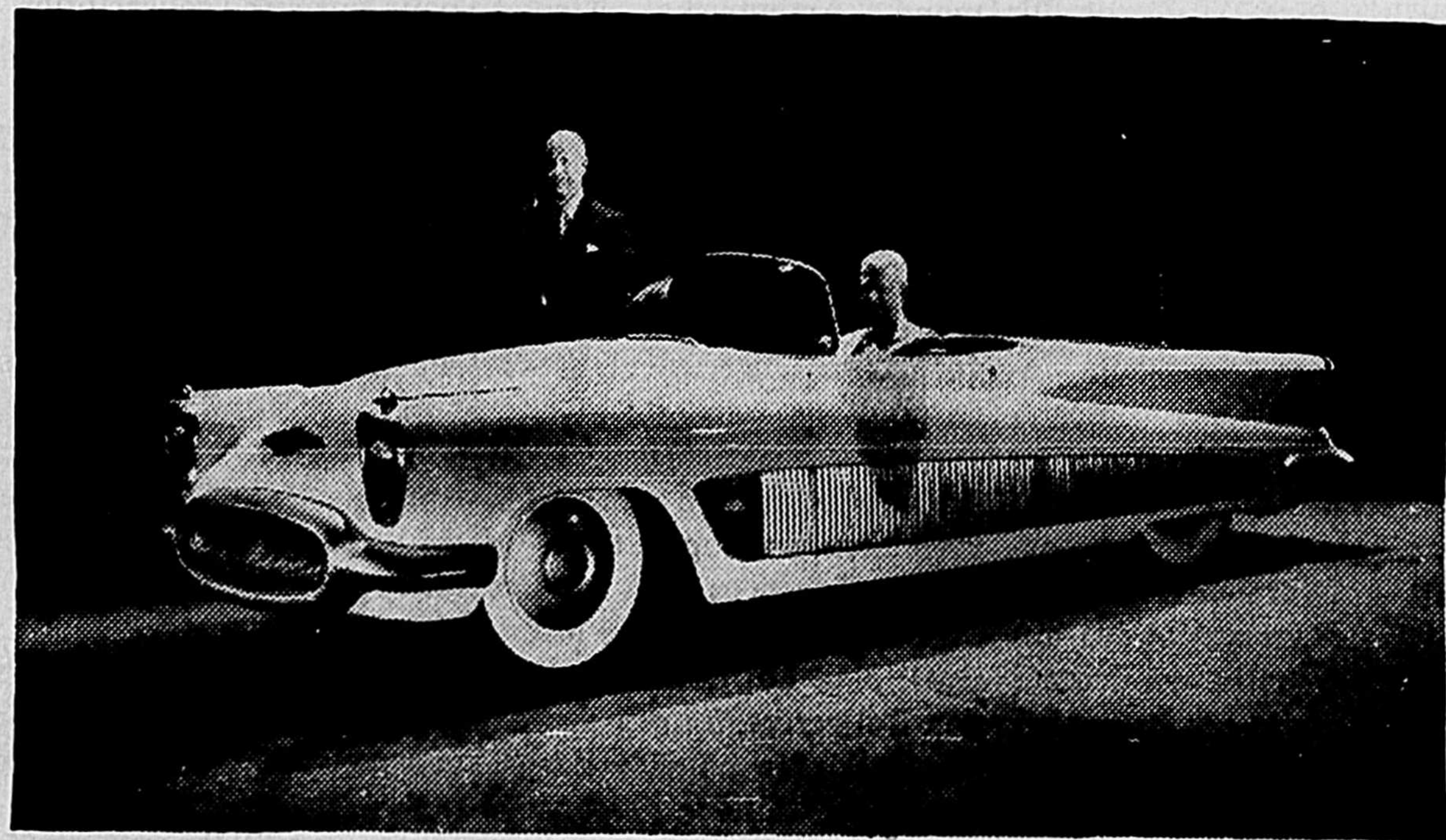
Voici la nouvelle voiture expérimentale BUICK-X P-300. Construite entièrement en aluminium, elle a une puissance de 200 chevaux et peut rouler à 150 milles à l'heure. Ce modèle complètement automatique sera mis sur le marché dès que les conditions se seront améliorées.
