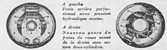
À gauche: Frein arrière perfectionné avec pression hydraulique accrue. À droite: Nouveau genre de frein de nous avant de la droite avec action deux-cylindres.
