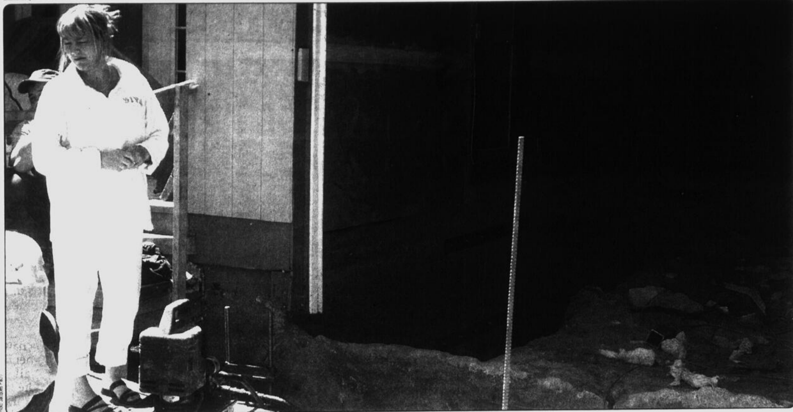
Avant de poser les pieux, des ouvriers ont creusé une fosse tout autour des trois murs extérieurs du garage de Danielle Gaudreau, ainsi qu'à l'intérieur du mur attenant à la maison.
