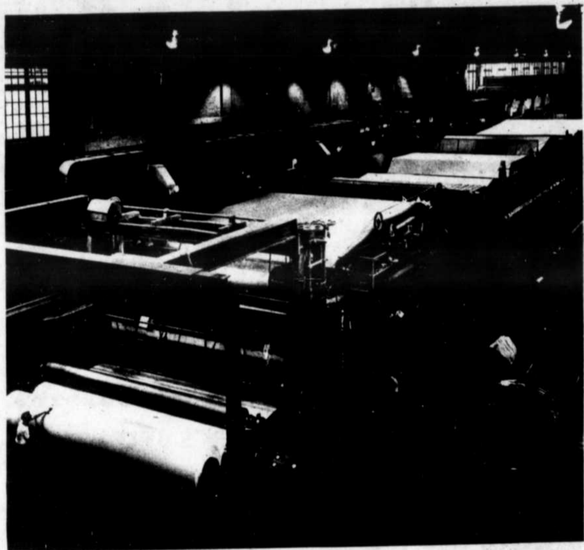
Deux des quatre machines actuellement en marche à l'usine de Gatineau. Toutes sont à peu près identiques. Celle que l'on voit ci-haut a une capacité quotidienne de production de 270 tonnes une largeur d'embobinage de 259 pouces.
