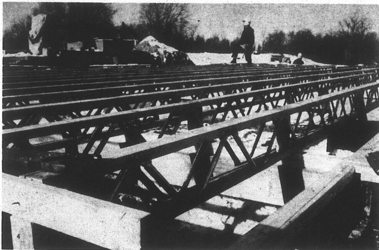
La poutrelle de plancher qui sera produite par la firme Romaro de St-Victor aura cet aspect.
