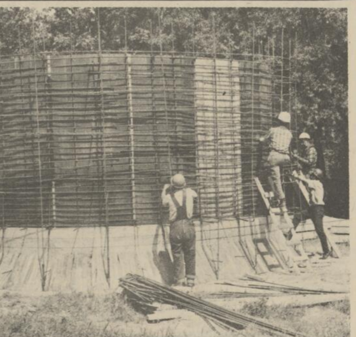
LES TRAVAUX DE CONSTRUCTION d'une usine de pompage dans la paroisse St-Jean l'Évangéliste progressent rapidement. En effet, des ouvriers ont terminé le montage des formes en vue de recevoir les milliers de tonnes de béton armé qui seront versées pour cet édifice. On sait que les travaux de construction du service d'égout et d'aqueduc de cette municipalité coûteront une somme de $1,100,000.
