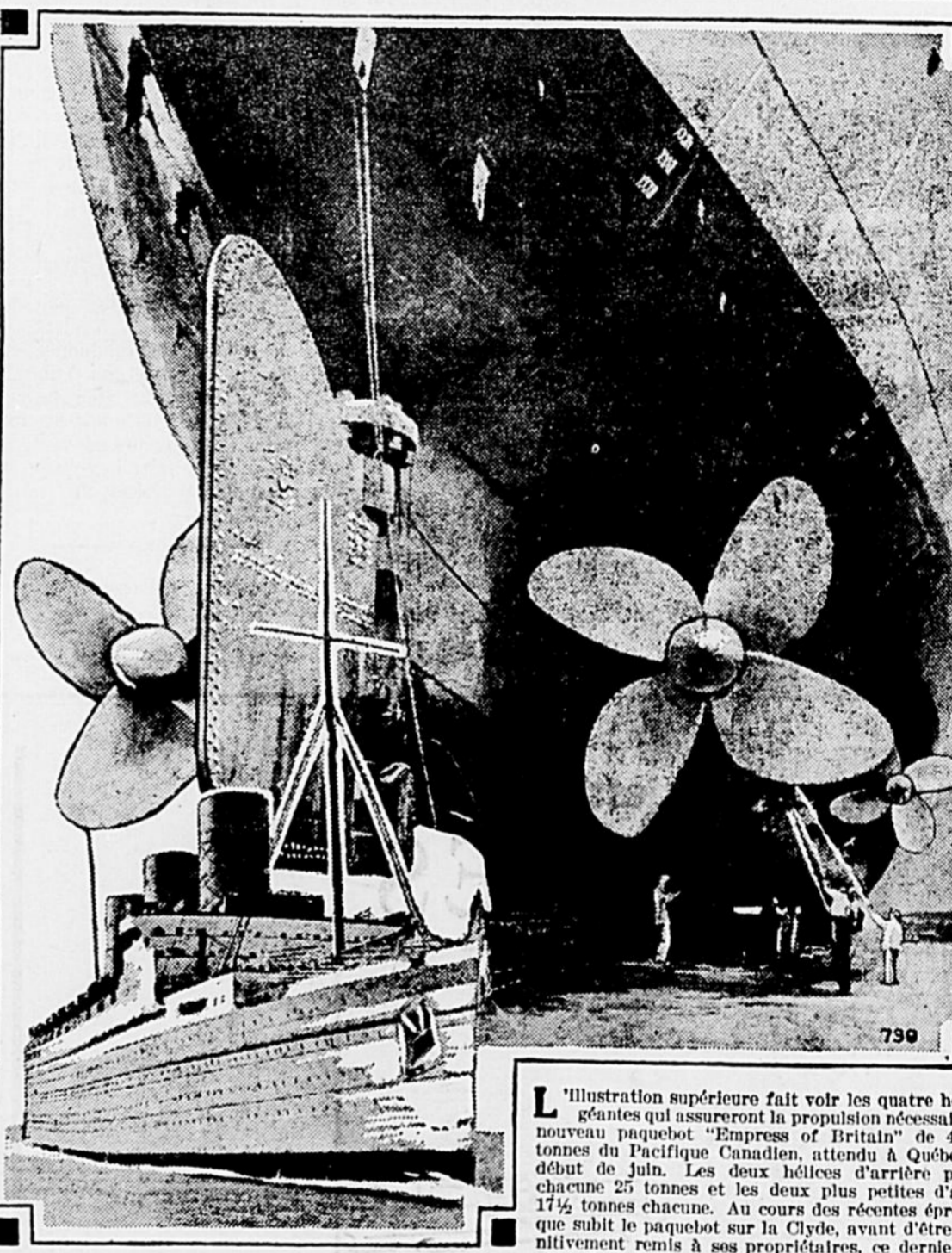
L'illustration supérieure fait voir les quatre hélices géantes qui assurent la propulsion nécessaire au nouveau paquebot "Empress of Britain" de 42,500 tonnes du Pacifique Canadien, attendu à Québec au début de juin. Les deux hélices d'arrière pèsent chacune 25 tonnes et les deux plus petites d'avant 17 1/2 tonnes chacune. Au cours des récentes épreuves que subit le paquebot sur la Clyde, avant d'être définitivement remis à ses propriétaires, ce dernier put atteindre une vitesse maximum de 25 1/2 nœuds sur le mille mesuré — On peut aussi voir sur la gravure le puissant gouvernail du super-paquebot, qui pèse 67 tonnes. A cet effet et quelques jours auparavant, une équipe d'hommes avait libéré la route des poteaux de téléphone. La vignette du bas montre l'"Empress of Britain" au cours de ses essais sur la Clyde, il y a quelques semaines. Le paquebot quittera Southampton le 27 mai et arrivera à Québec cinq jours plus tard.
