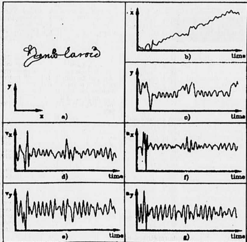
Reconnaissance de signature: traces graphiques d'une signature. Les graphiques b et c (en haut à droite) correspondent à la position du crayon électronique; les graphiques d et e (en bas à gauche) indiquent la vitesse de l'écriture; les graphiques f et g (en bas à droite) témoignent de l'accélération du mouvement au cours de la signature.
