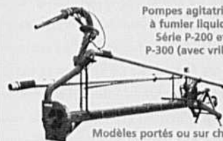
Modèles portés ou sur châssis porteur avec 2 ou 4 roues.
