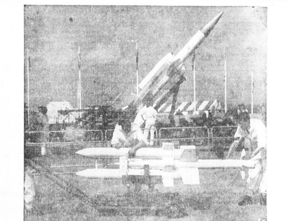
LA GRANDE-BRETAGNE A SES MISSILES: Les hommes de la R. A. F. préparent un "Fireflash", engin teleguidé air-air, pour une exposition à Farnborough (Angle-
