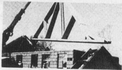
On complète ensuite le charpentage de la couverture en faisant la pose de fermes de couverture et du contreplaqué de 1/2" d'épaisseur contrairement au contreplaqué de 3/8" utilisé encore sur la construction ordinaire. Le revêtement extérieur n'est pas inclus avec le kit de maison.
