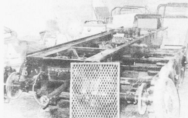
Le "frame", la structure du "Ski Dozer" repeinte et dans un état de recevoir la cabine, le moteur et les chenilles. (Photo Geles)
