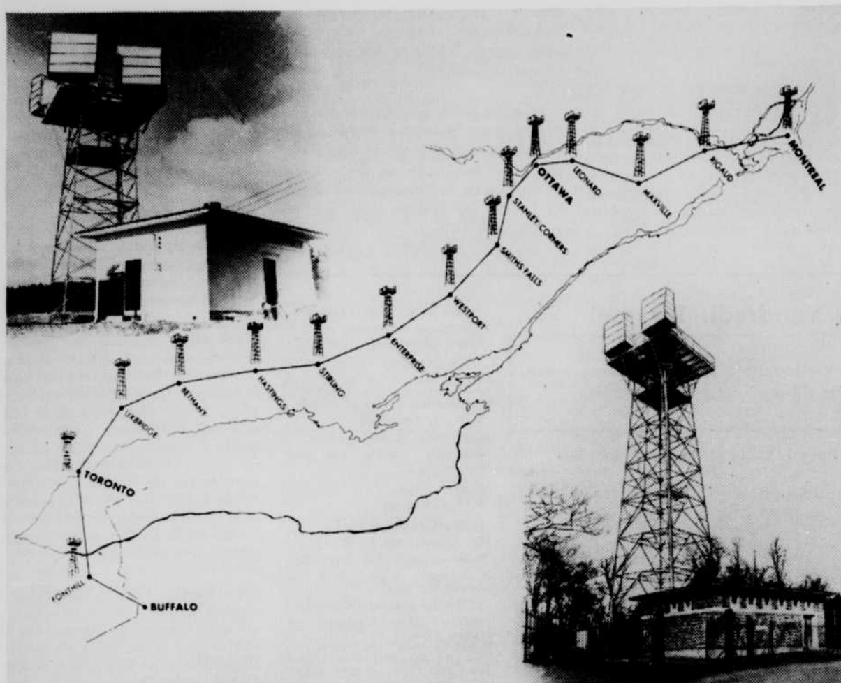
Carte du réseau de télévision de Radio-Canada avec ses relais à ondes micrométriques qui ont été érigés par la Compagnie de téléphone Bell. En bas, à droite, le pylône terminus de Montréal, qui a été érigé sur le mont Royal. On aperçoit à l'arrière-plan l'antenne de CBFT. En haut, à gauche, l'une des 13 stations de relais entre Montréal, Ottawa et Toronto.
