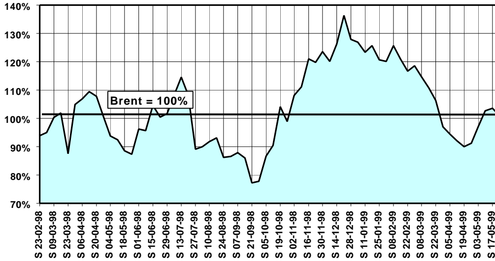
Graphique n°2 Ratio Huile n°6, 1,5 % de soufre versus prix du Brent (Prix du Brent = 100)
