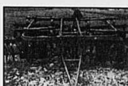
Herse JD 115, 44 roulettes, herse JD 620, 36 disques. PSD
