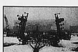
1 cultivateur 27 pds Allis Chalmers, dent en C, pointes de 4.5 pouces. PSD
