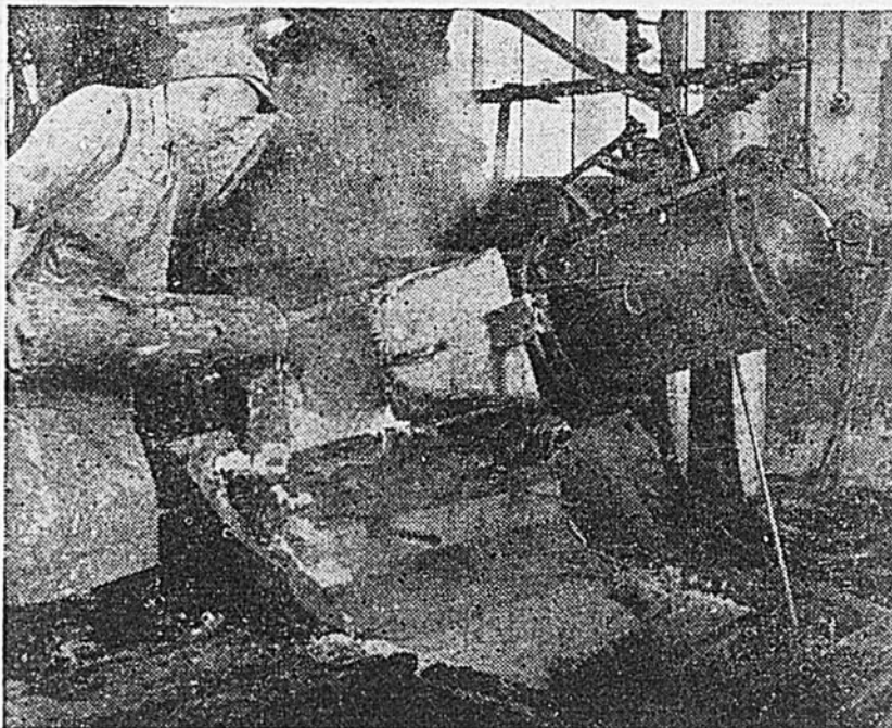
Les billots écorcés sont introduits dans les broyeurs; de puissants ressorts y pressent le bois contre des meules en grès qui tournent rapidement; le bois en sort en menus copeaux.
