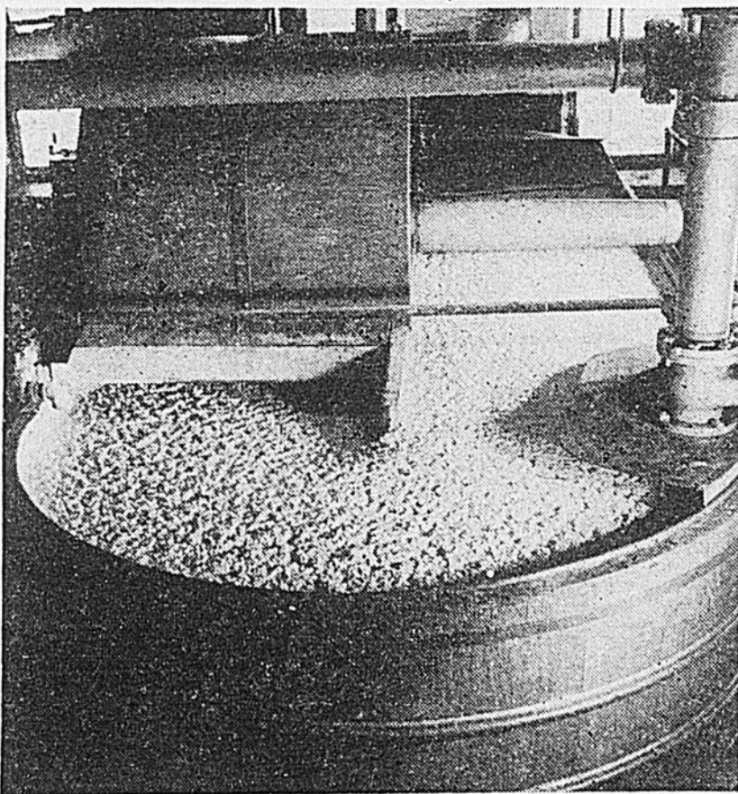
Les copeaux baignent dans l'eau et sont soumis à des secousses. Peu à peu les fibres du bois se gonflent, s'enchevêtrent et forment une pâte qui s'écoule sur des tamis. C'est la pâte mécanique qui entre dans la composition du papier à journal à raison de 85 pour 100.
