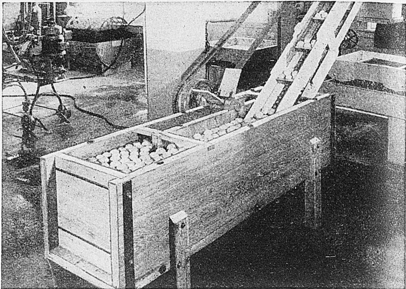
Bien que cette photographie appartienne plutôt au domaine industriel qu'à l'entreprise domestique on y observe cependant quelques facteurs très importants pour la fabrication d'un bon cidre. On remarquera que les pommes sont fraîches et que le procédé de manutention s'accomplit avec propreté.
