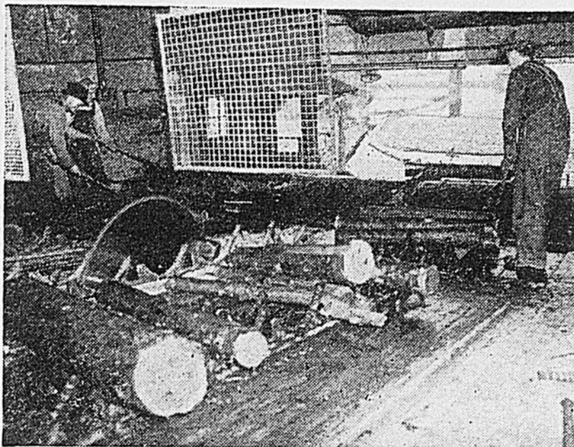
Les billots sont ensuite conduits vers les écorceurs formés d'une succession de couteaux qui degarnissent le bois par écorçage progressif.
