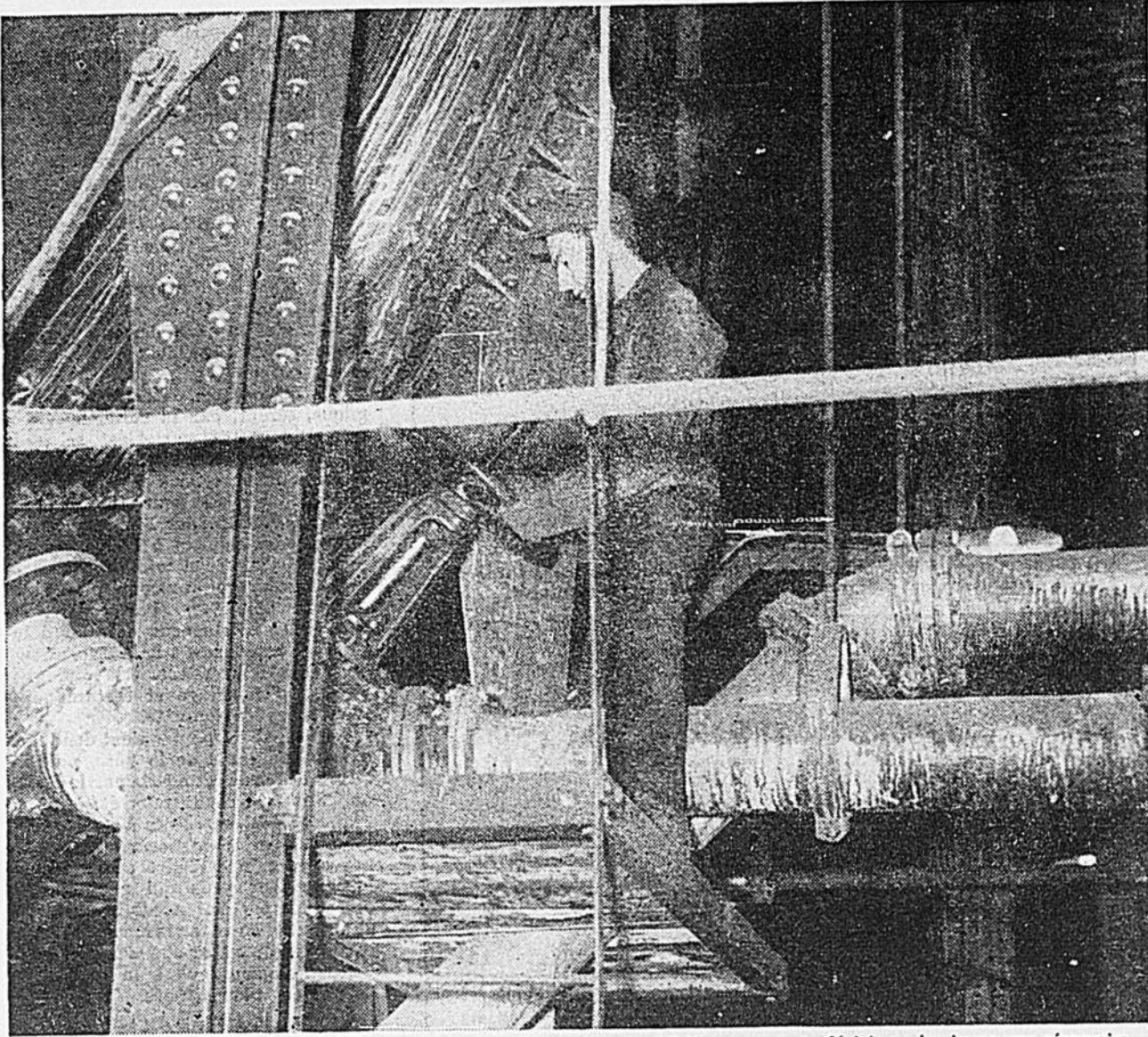
La pâte chimique s'obtient par l'action d'un acide sur le bois réduit en copeaux. Voici un des immenses réservoirs qui contiennent l'acide sulfite. La pâte traitée à l'acide sulfite est mêlée à la pâte mécanique en des proportions de 15 pour 100 pour le papier à journal et davantage dans les papiers à écrire.
