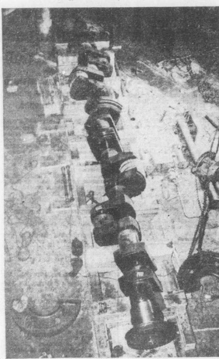
Cette curieuse pièce de métal, reposant dans la cale du "Beaverbrae", du Pacifique Canadien, est un arbre-vilebrequin, pesant 13 tonnes et demie, que l'on est en train d'installer sur le navire en la cale sèche des chantiers Vickers, de Montréal. Lors des réparations que l'on avait fait subir à l'ancien cargo allemand, aux chantiers de Sorel, on s'était rendu compte que la pièce avait besoin d'être changée, mais la fabrication a nécessité un certain temps et le bateau a été mis en service en attendant que l'arbre soit construit à Erie, Pennsylvanie. La mise en place de cette pièce nécessitera le déplacement de près de 200 tonnes de machinerie du "Beaverbrae". On a aussi été forcé de percer la paroi d'acier séparant la cale de la chambre des machines. (photo Pacifique Canadien)
