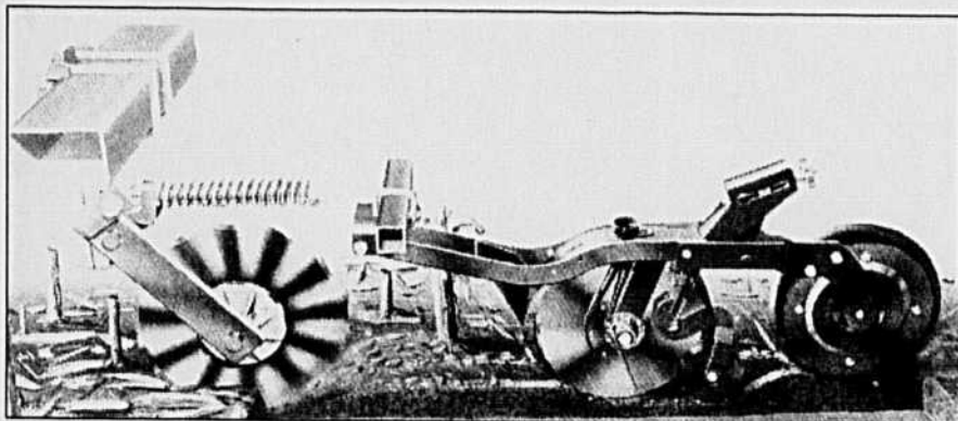
Principe de fonctionnement d'un semoir direct
