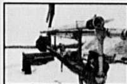
Pompe à lagune Rovibec, 25' hydraulique, 1 an d'usage, très propre. PSD
