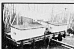
Planteur à maïs Cyclo 900, 6 rgs, avec vis à engrais
