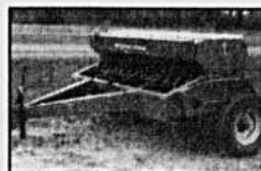
Semoirs à céréales 8 à 12' largeur, plusieurs marques, modèles, très beau choix, à partir de 800 $
