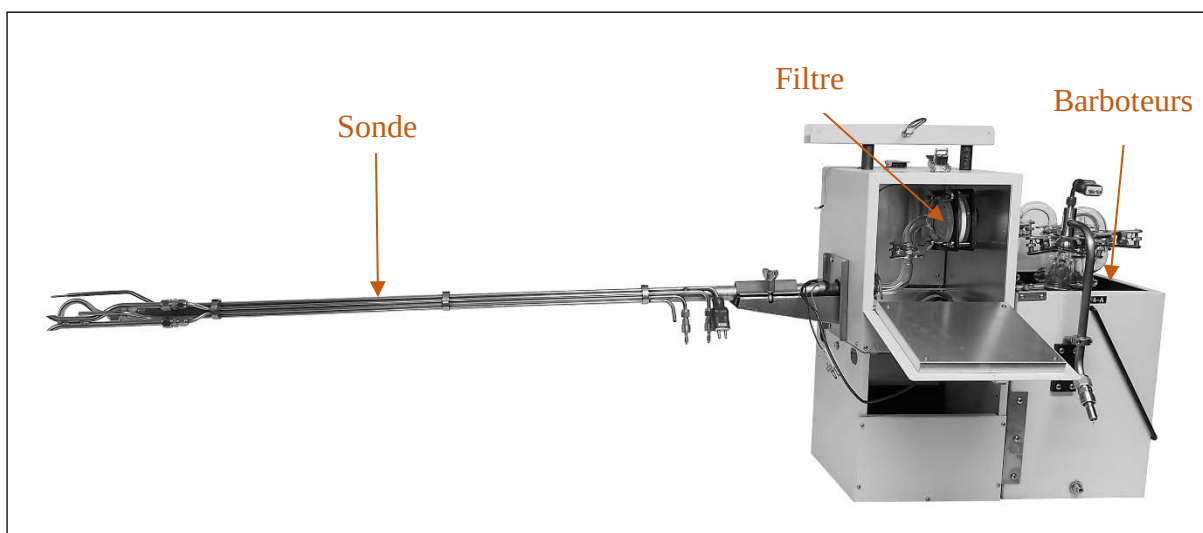
Figure 1 : Exemple de dispositif d'échantillonnage pour une méthode manuelle utilisant un filtre et des barboteurs
