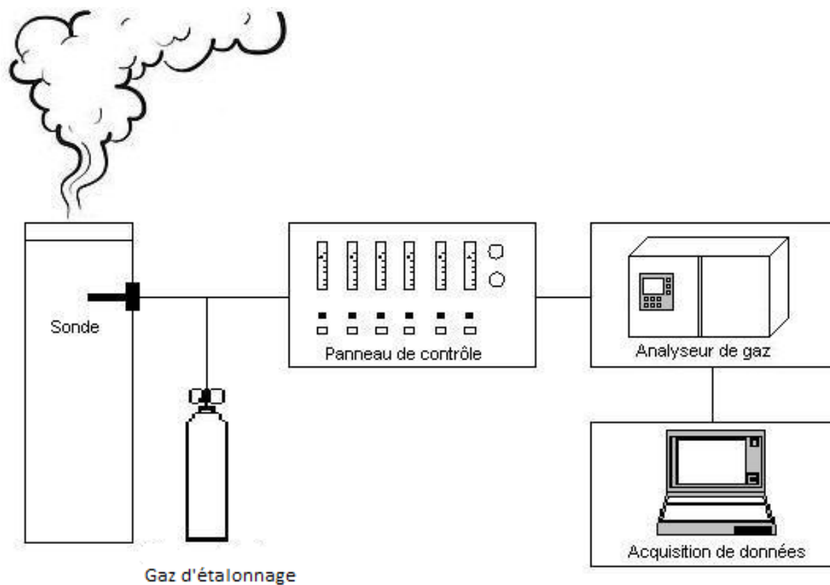
Shéma 1 : SMEC extractif
