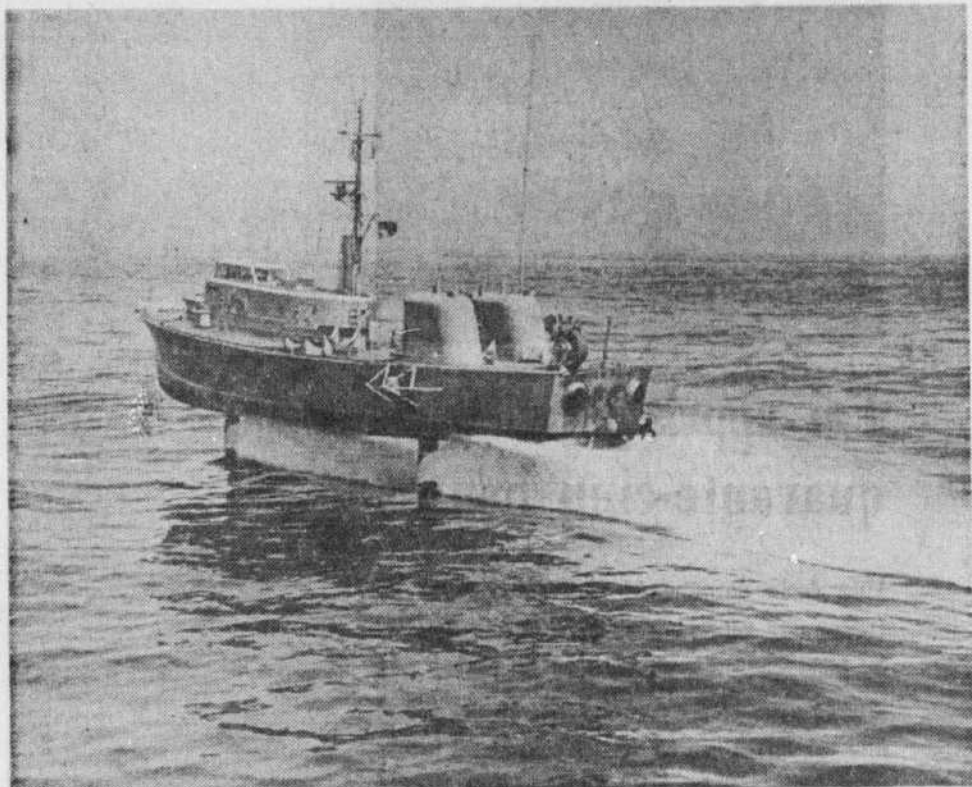
NAVIRE-BOLIDE À L'ESSAI — La marine américaine a récemment fait subir les premiers essais à l'unique hydrofoile actuellement en opération. C'est sur la côte nord-ouest, dans l'État de Washington, que le navire s'est "élevé" au-dessus de vagues de plus de cinq pieds,
