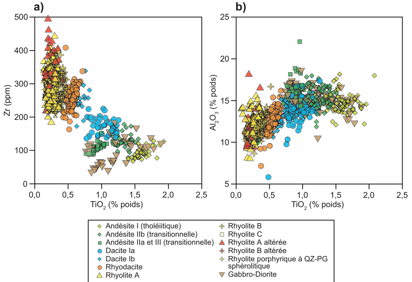
FIGURE 5 - a) Diagramme Zr versus TiO_2 ; b) diagramme Al_2O_3 versus TiO_2 pour les différentes roches volcaniques et intrusives du secteur à l'étude.
