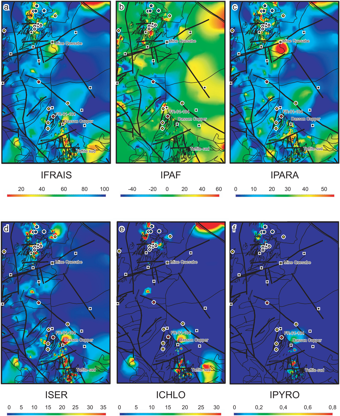
FIGURE 7 - Cartes de contours des indices d'altération des minéraux normatifs (Piché et Jébrak, 2004) du secteur étudié : a ) IFRAIS (indice des minéraux frais); b ) IPAF (indice de la perte au feu); c ) IPARA (indice de la paragonite hydrothermale); d ) ISER (indice de la séricite hydrothermale); e ) ICHLO (indice de la chlorite hydrothermale); et f ) IPYRO (indice de la pyrophyllite).
