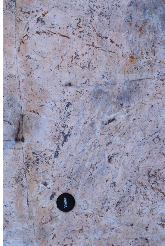
PHOTO 3 - Rhyolite A à structure d'écoulement laminaire hématisée, albitisée avec magnétite et pyrite disséminées. Indice Buffam, Affleurement 04-CD-1091 (UTM NAD 83, zone 17: 632290E, 5347924N).
