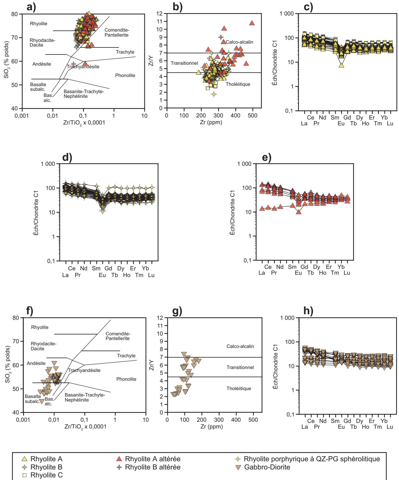
FIGURE 6 - a) et f) diagrammes de Winchester et Floyd (1977), b) et g) diagrammes d'affinité magmatique \text{Zr}/\text{Y} versus \text{Zr} (champs définis par Barrett et MacLean, 1999); c) d) e) h) diagrammes des éléments des terres-rares (normalisés par rapport à la chondrite C1 de McDonough et Sun, 1995) pour les rhyolites et les diorites-gabbros du secteur à l'étude.
