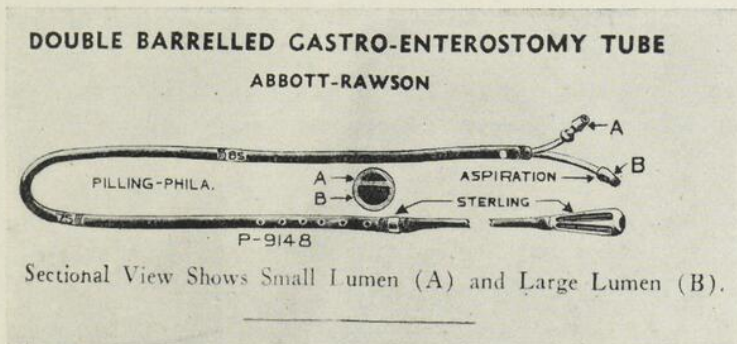
Fig. 3. — Tube d'Abbott-Rawson à double lumière.
