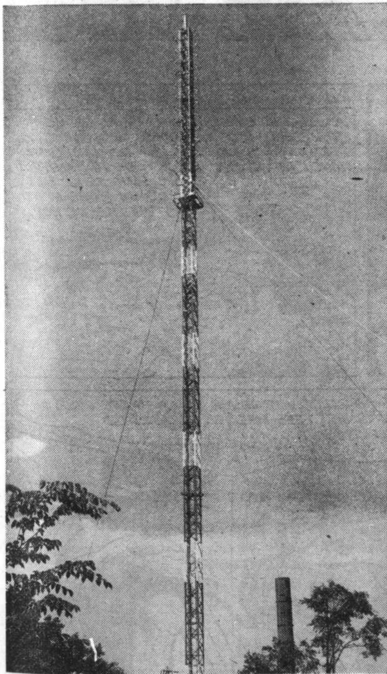
La tour supportant les antennes des postes de CBOT et CBOFT est le plus récent point de repère à Westboro, dans la banlieue d'Ottawa. S'élevant 488 pieds au-dessus du sol, la tour loge l'antenne de 18 pieds de CBOFT, canal 9, (complètement au haut), un guide d'ondes à quatre ouvertures et l'antenne à 12 sections de haute puissance de CBOT, canal 4, dont on peut voir les arêtes sur les côtés. Pour juger de la hauteur de la nouvelle tour, comparez avec l'antenne temporaire, au premier plan à droite, qui mesure 75 pieds de haut.
